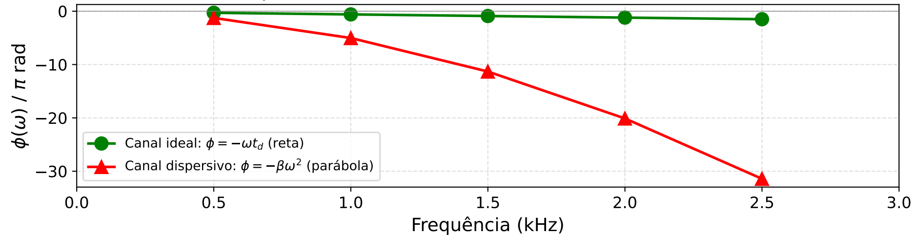
Espectro de Fase — Linear (reta) vs Não-linear (curva)
