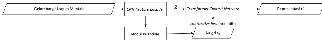
Gambar 2.3 Arsitektur Wav2Vec2
