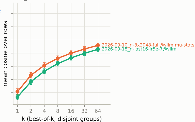
cos_centred
