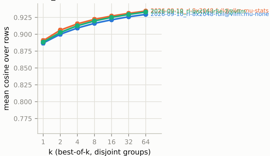
cos_raw
