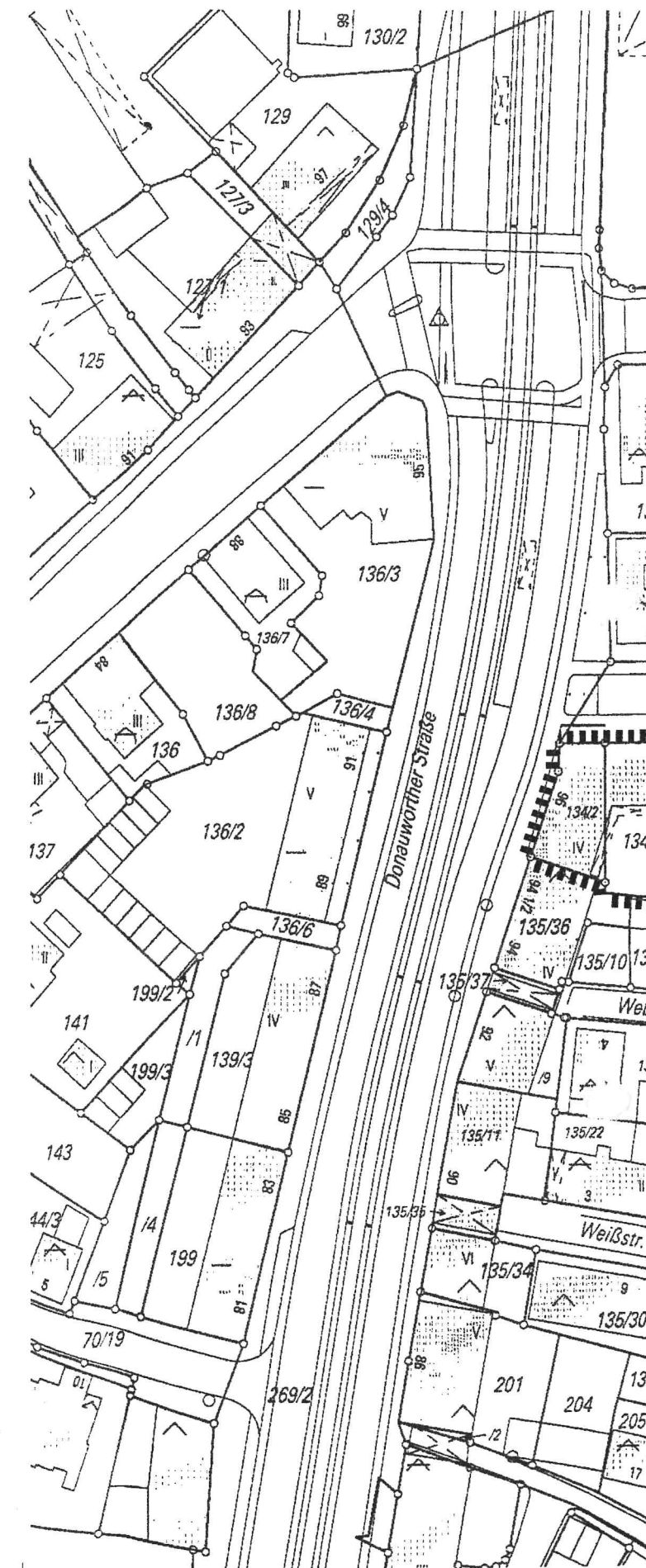
Lageplan M 1:10000
