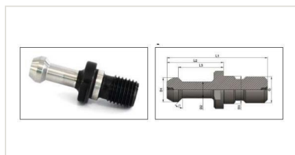
MAS 403 BT DIN ISO 7388-3
