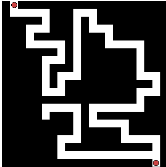
step 25
