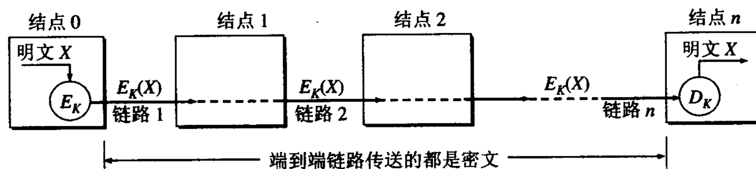
图 7-15 端到端加密
