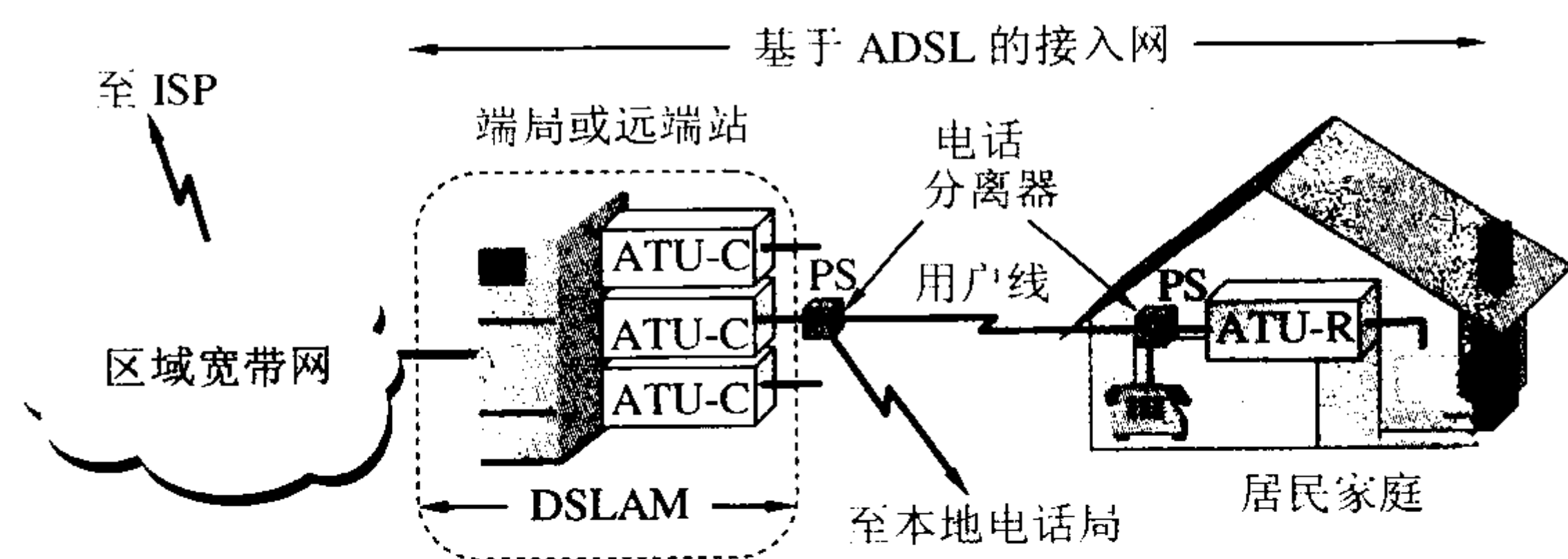
图 2-20 基于 ADSL 的接入网的组成
