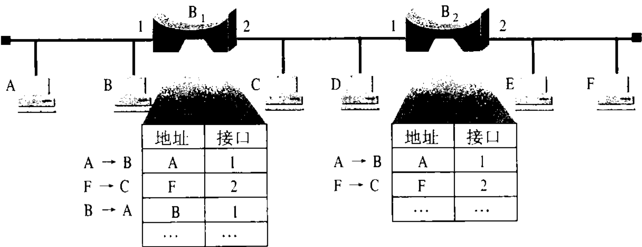
图 3-28 网桥的自学习和转发过程
