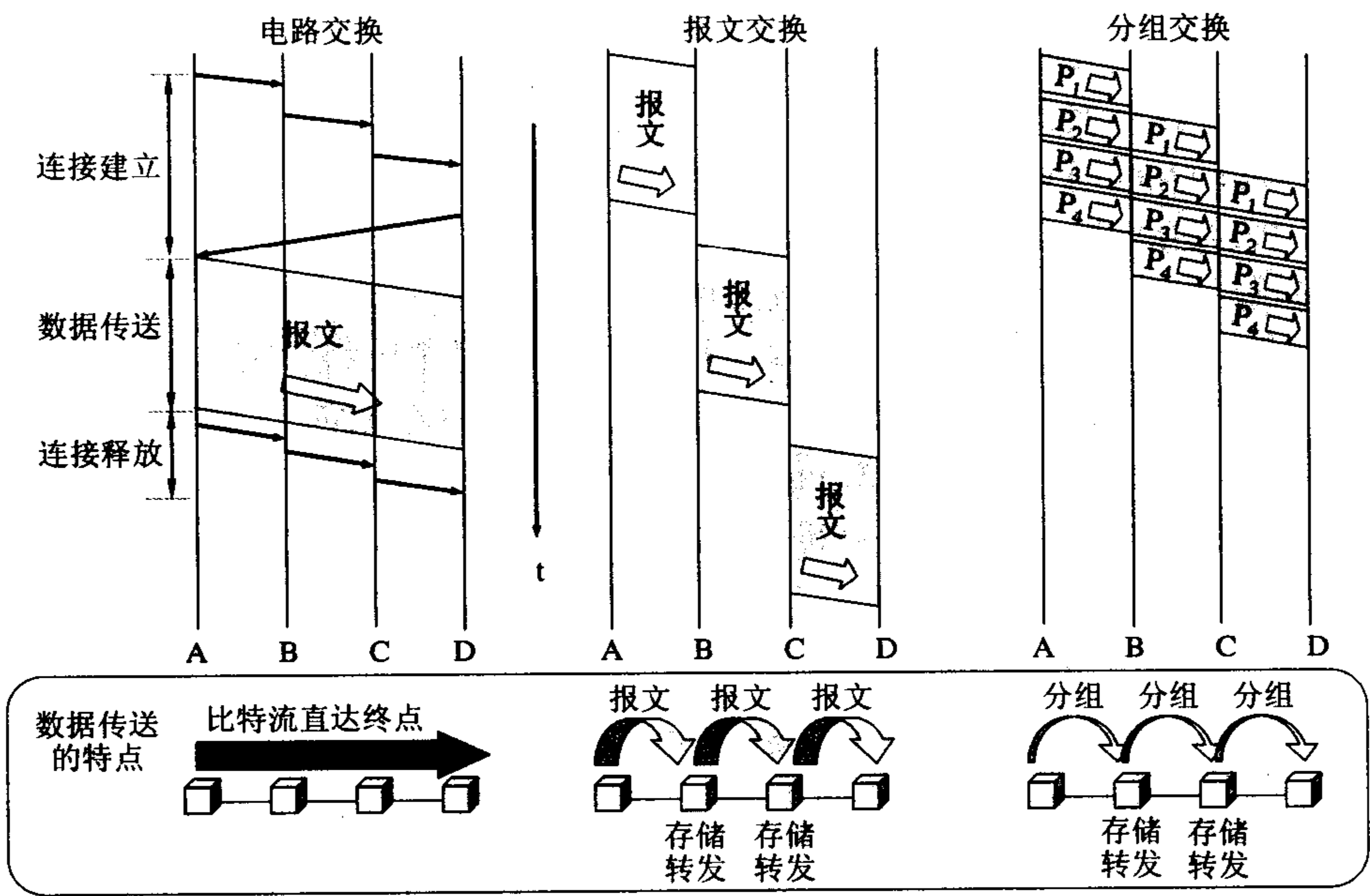
图 1-12 三种交换的比较：电路交换；报文交换；分组交换，P 1 ~P 4 表示 4 个分组
