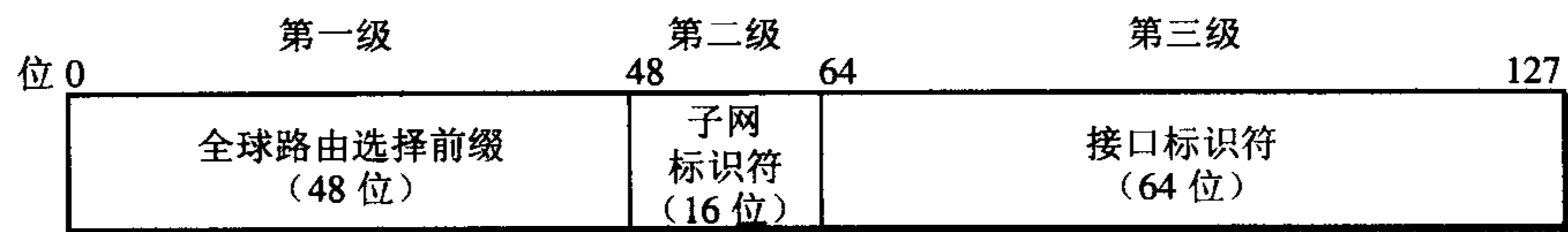
图 10-7 IPv6 单播地址的等级结构
