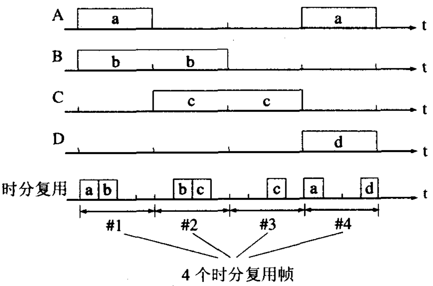
图 2-14 时分复用可能会造成线路资源的浪费
