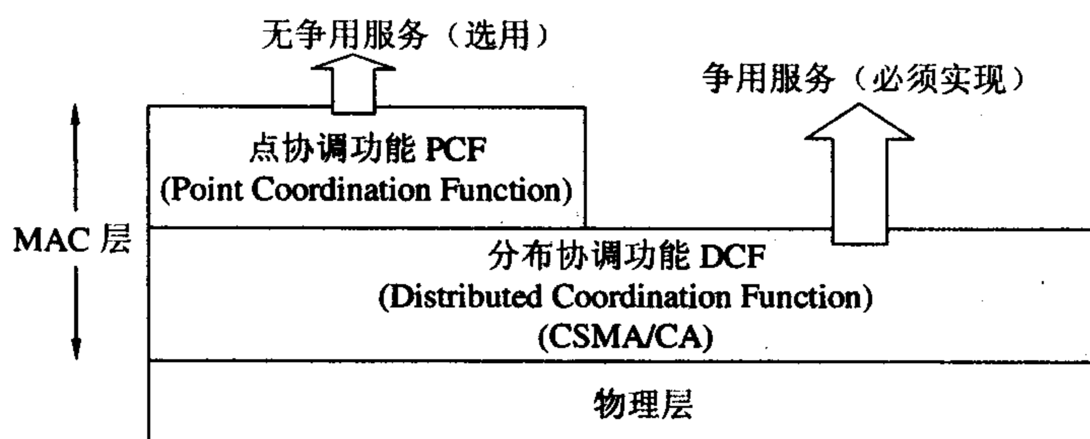
图 9-5 802.11 的 MAC 层
