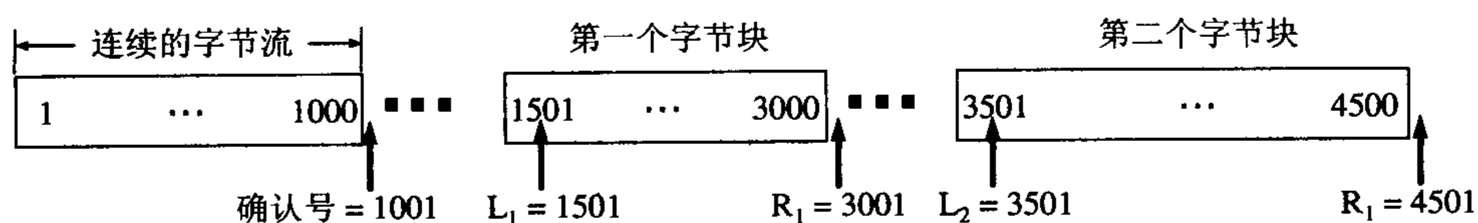
图 5-21 接收到的字节流序号不连续
