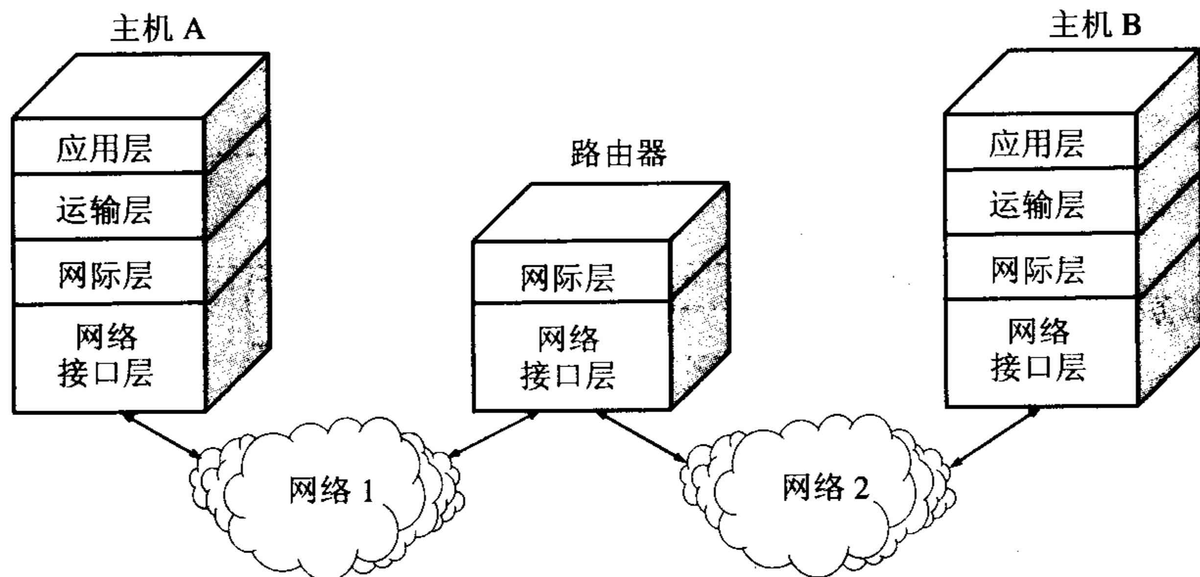
图 1-20 TCP/IP 四层协议的表示方法举例
