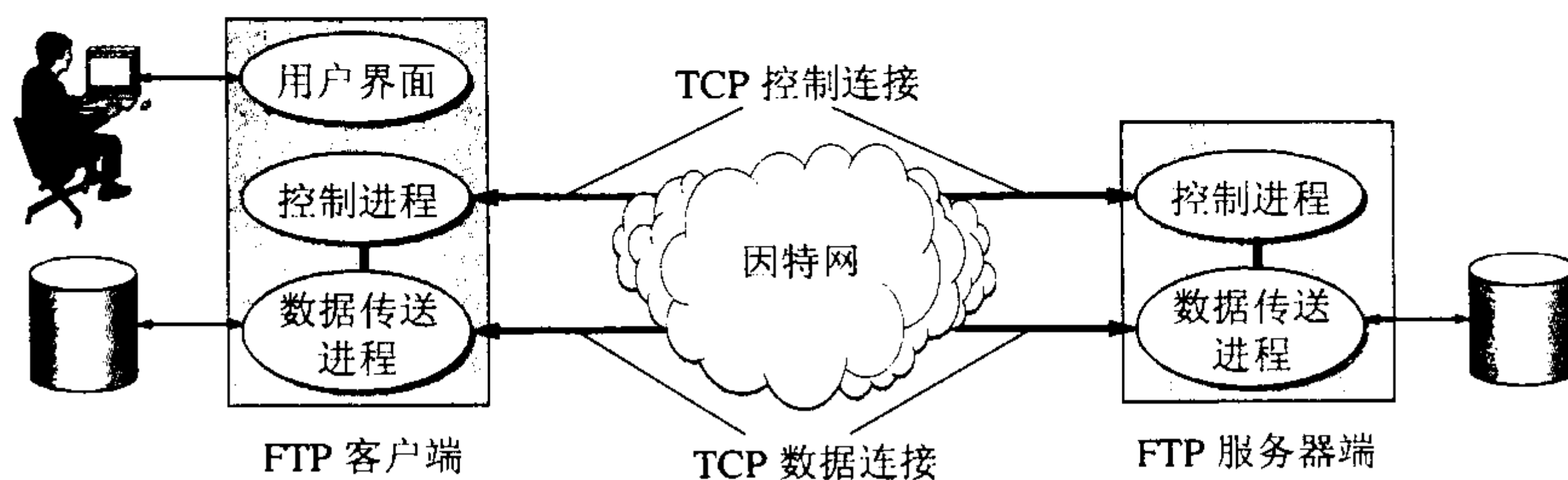
图 6-6 FTP 使用的两个 TCP 连接
