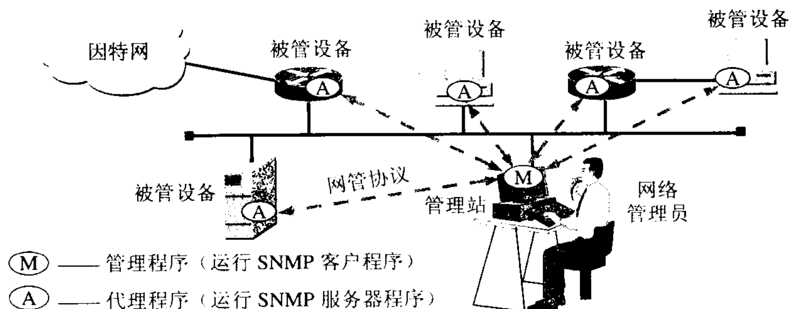
图 6-22 网络管理的一般模型
