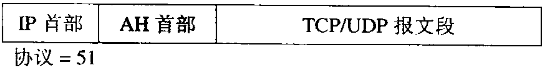
图 7-12 AH 首部在安全数据报中的位置
