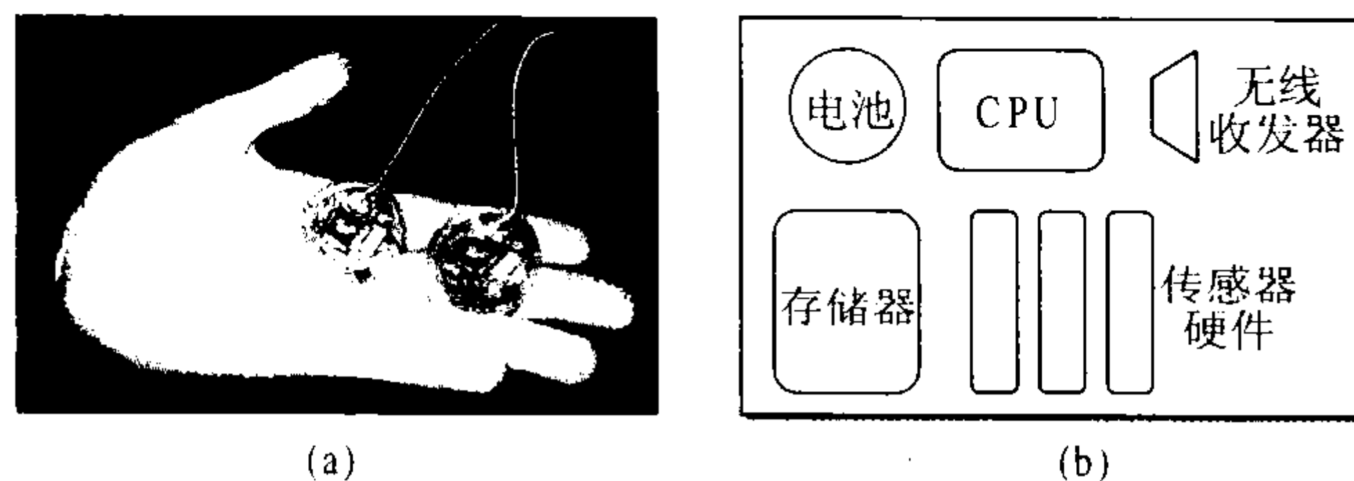
图 9-3 传感器结点的形状(a)和组成(b)
