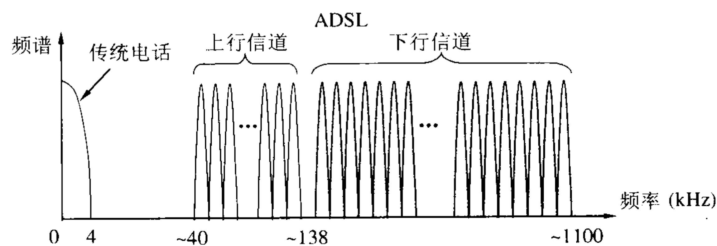
图 2-19 DMT 技术的频谱分布
