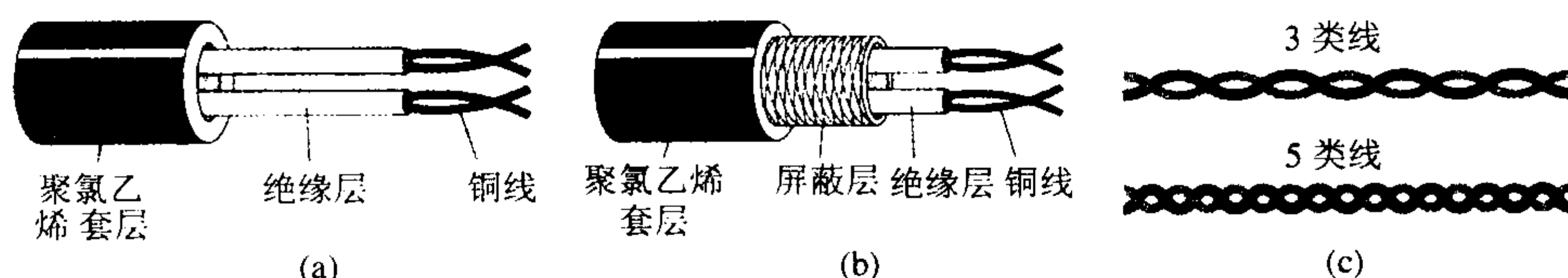
图 2-4 双绞线的示意图：(a) 无屏蔽双绞线；(b) 屏蔽双绞线；(c) 不同的绞合度的双绞线
