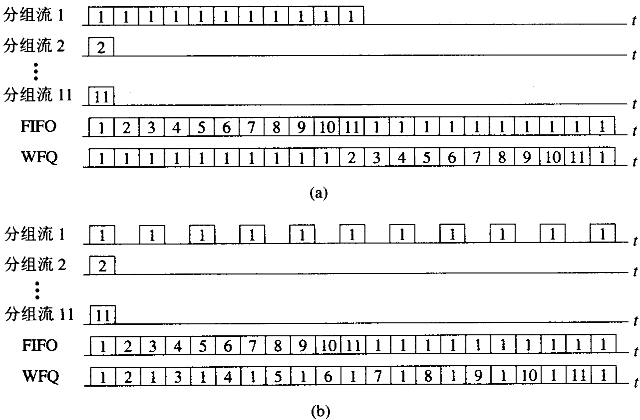
图 8-20 WFQ 与 FIFO 的比较
