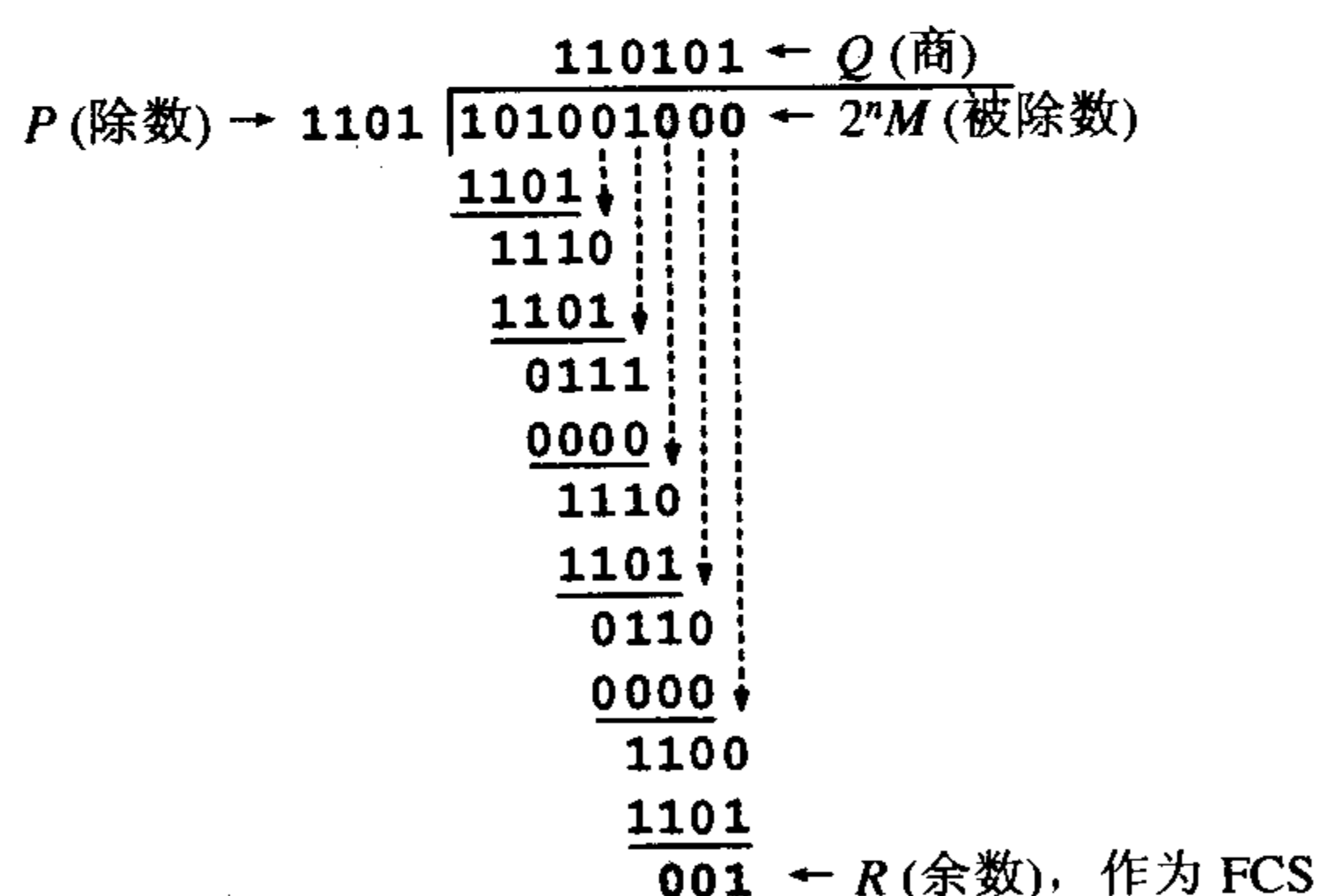
图 3-8 说明循环冗余检验原理的例子
