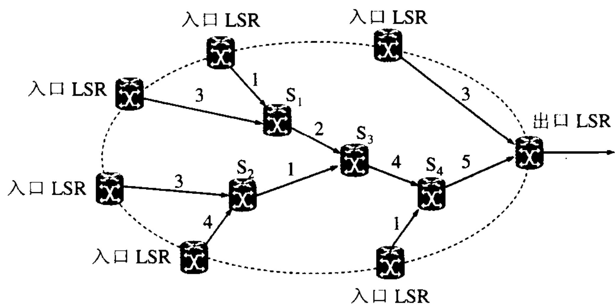
图 10-13 应用流聚合到出口 LSR
