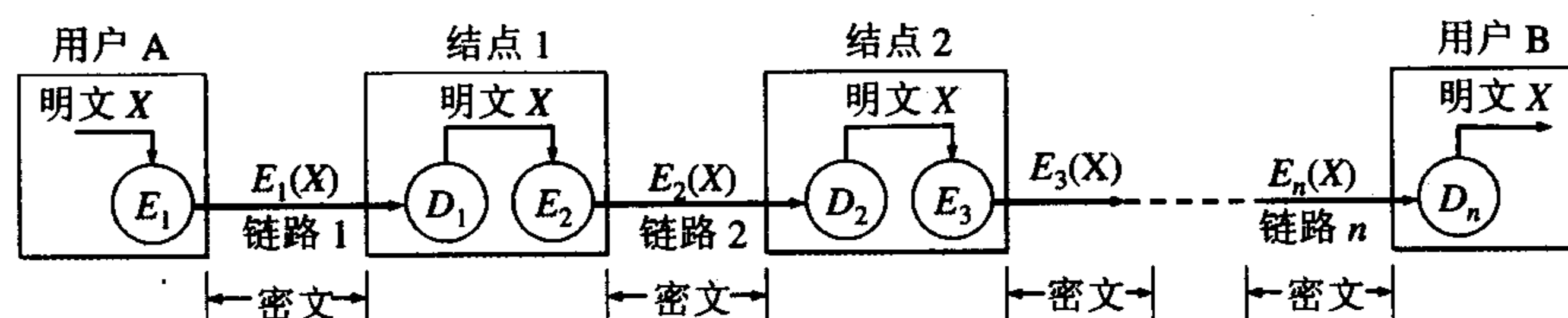
图 7-14 链路加密
