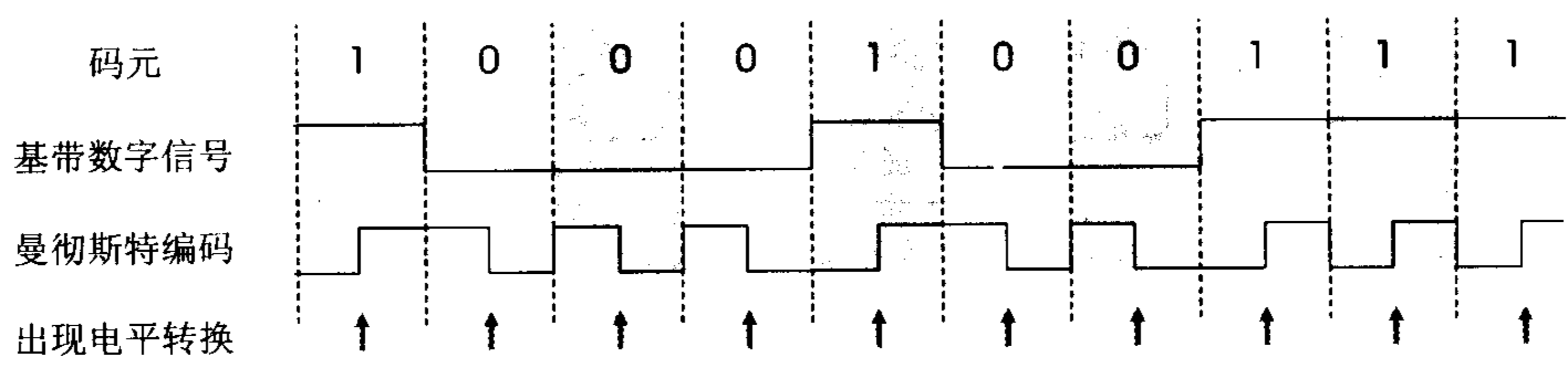
图 3-16 曼彻斯特编码
