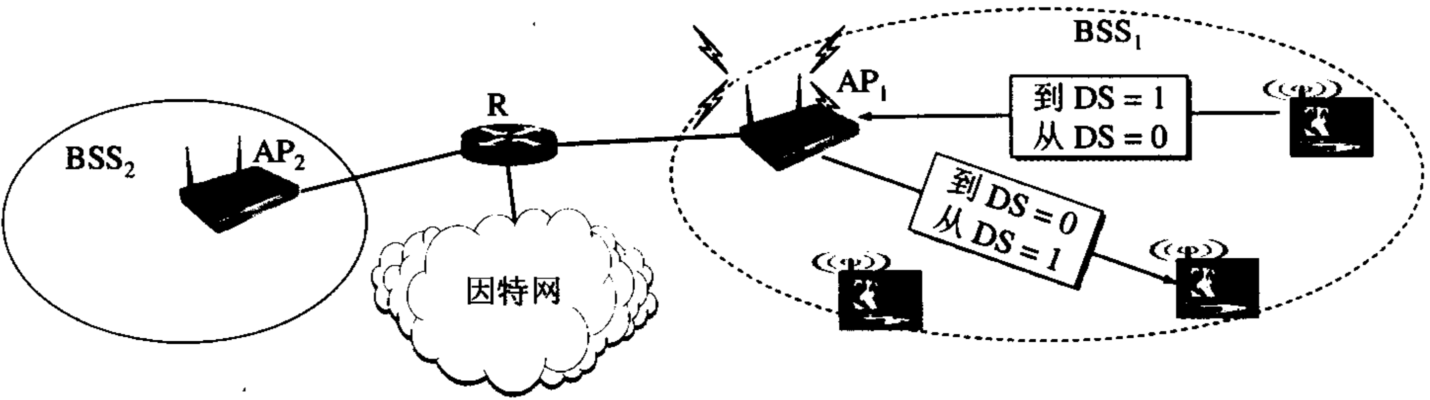
图 9-11 A 向 B 发送数据帧必须先发送到接入点 AP 1
