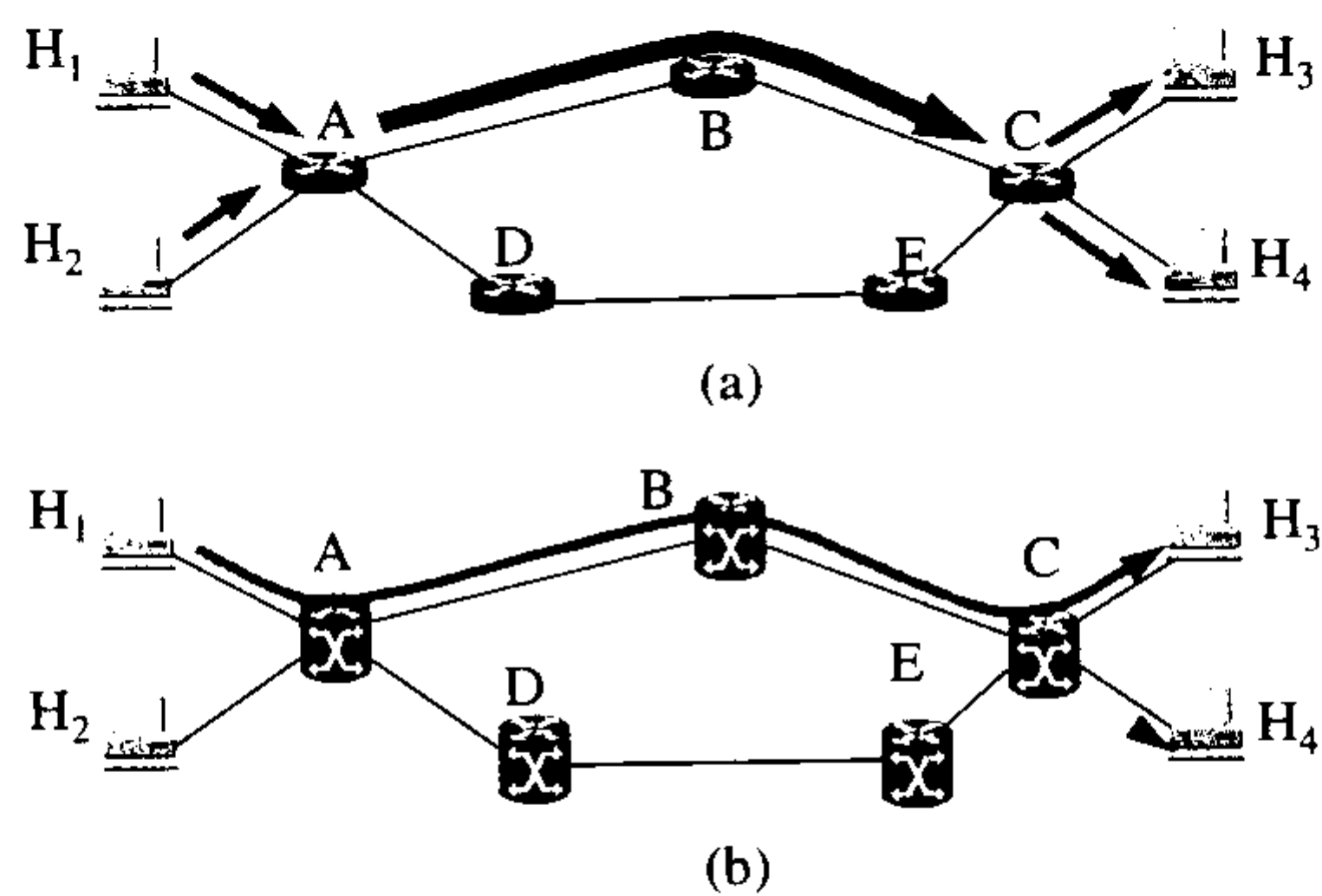
图 10-14 FEC 用于负载平衡
