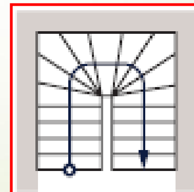
Escalier à double quartier tournant
