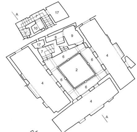
Niveau shin (Etage)
