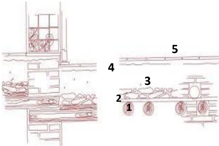
Planchers des maisons de la Casbah
