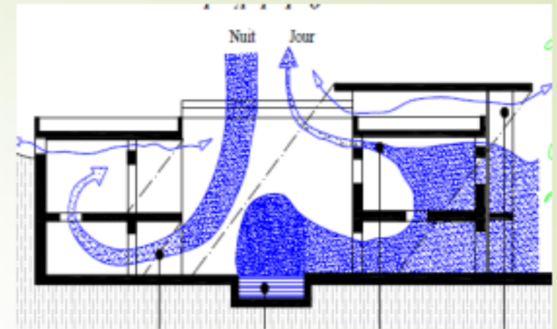
schéma de fonctionnement climatique d'un patio Source: chabi med
