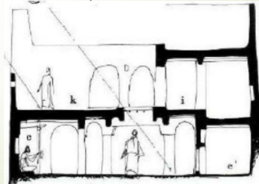
Patio adapté aux conditions climatiques Source André Ravéau
