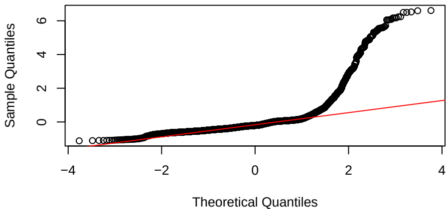
Q-Q Plot de Residuales
