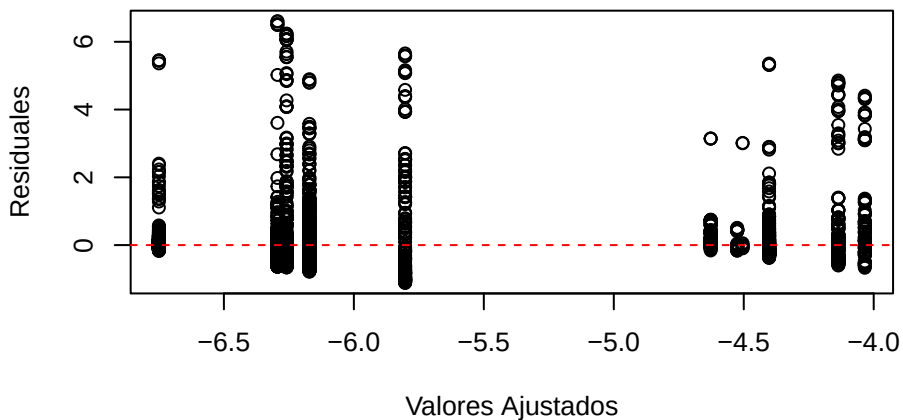
Residuales vs Valores Ajustados
