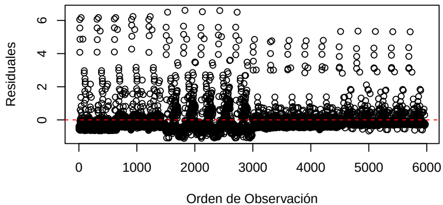
Residuales vs Orden
