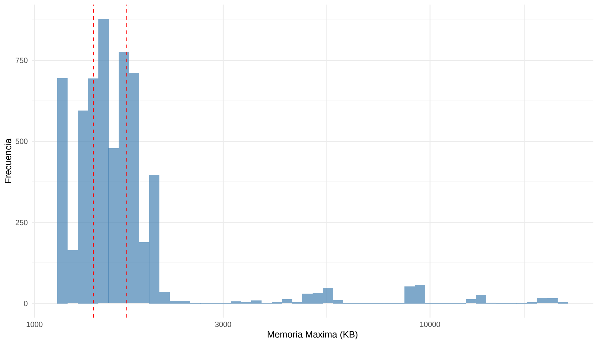
Distribucion del Uso de Memoria (max_mem_kb)
