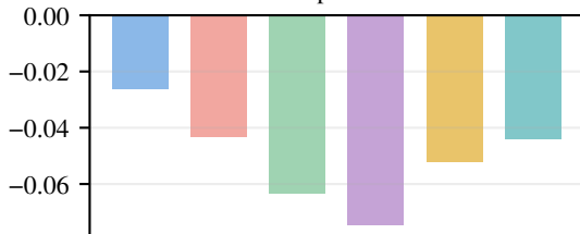
Map mAP
