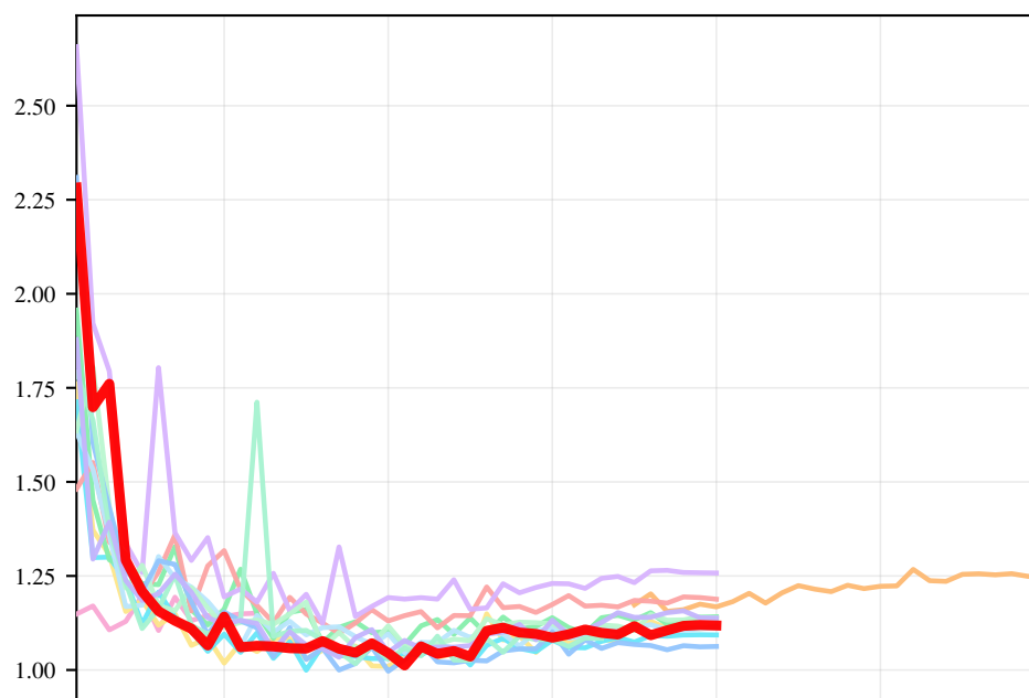
Motion FDE
