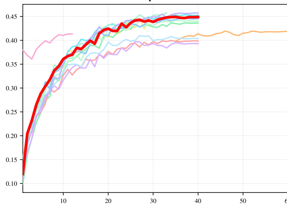
Map mAP
