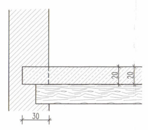
AUFLAGERNISCHEN AN1 M 1:25 32* AUSF.
