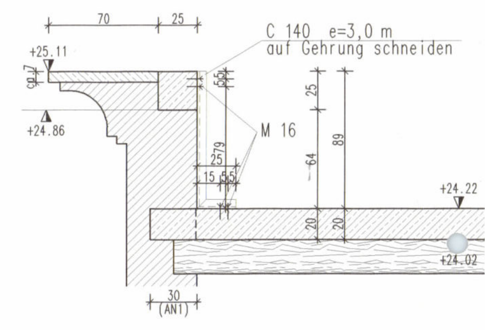
STB ROST 25/25 ÜBER GANZE LÄNGE UK=+24,86 OK=+25,11
