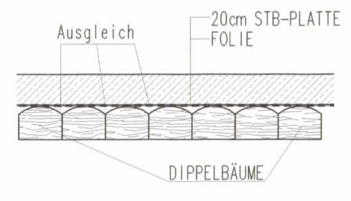
PLATTENQUERSCHNITT M 1:25
