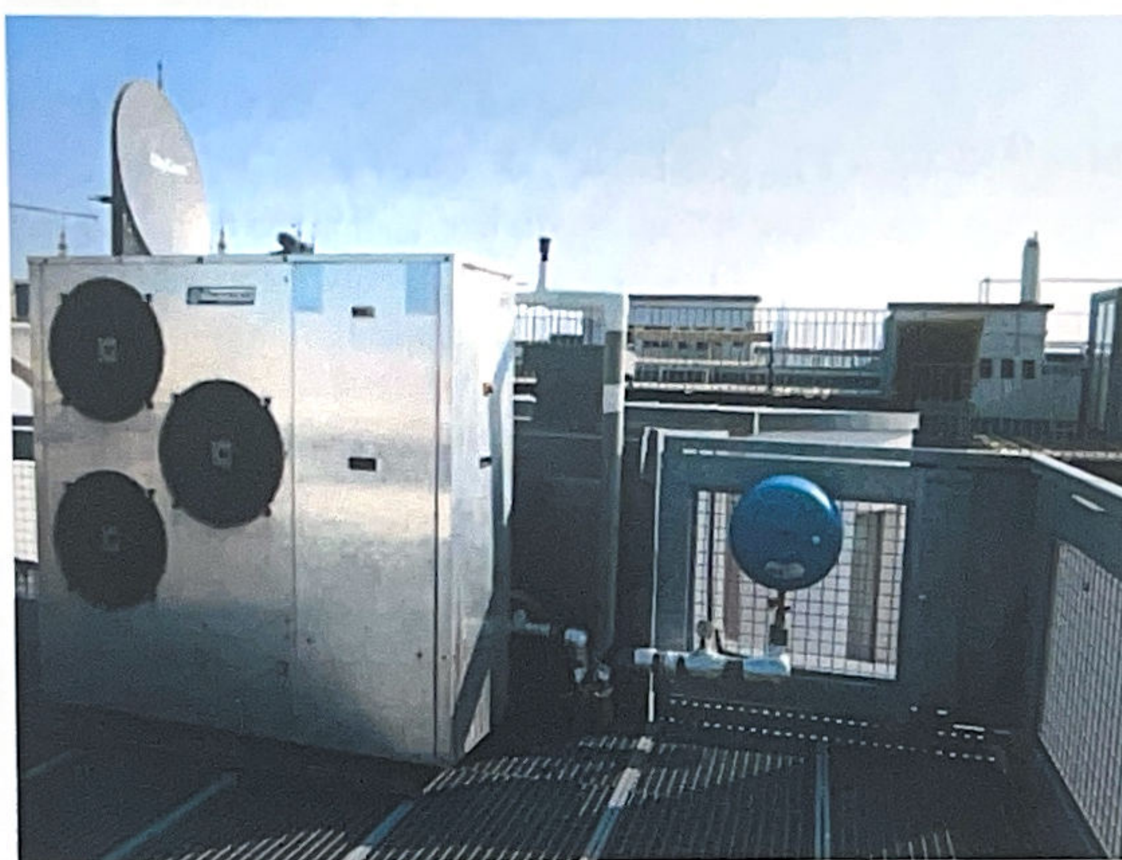
Abbildung 4: Kälteanlage am Dach des Hauses Landesgerichtsstr. 6
