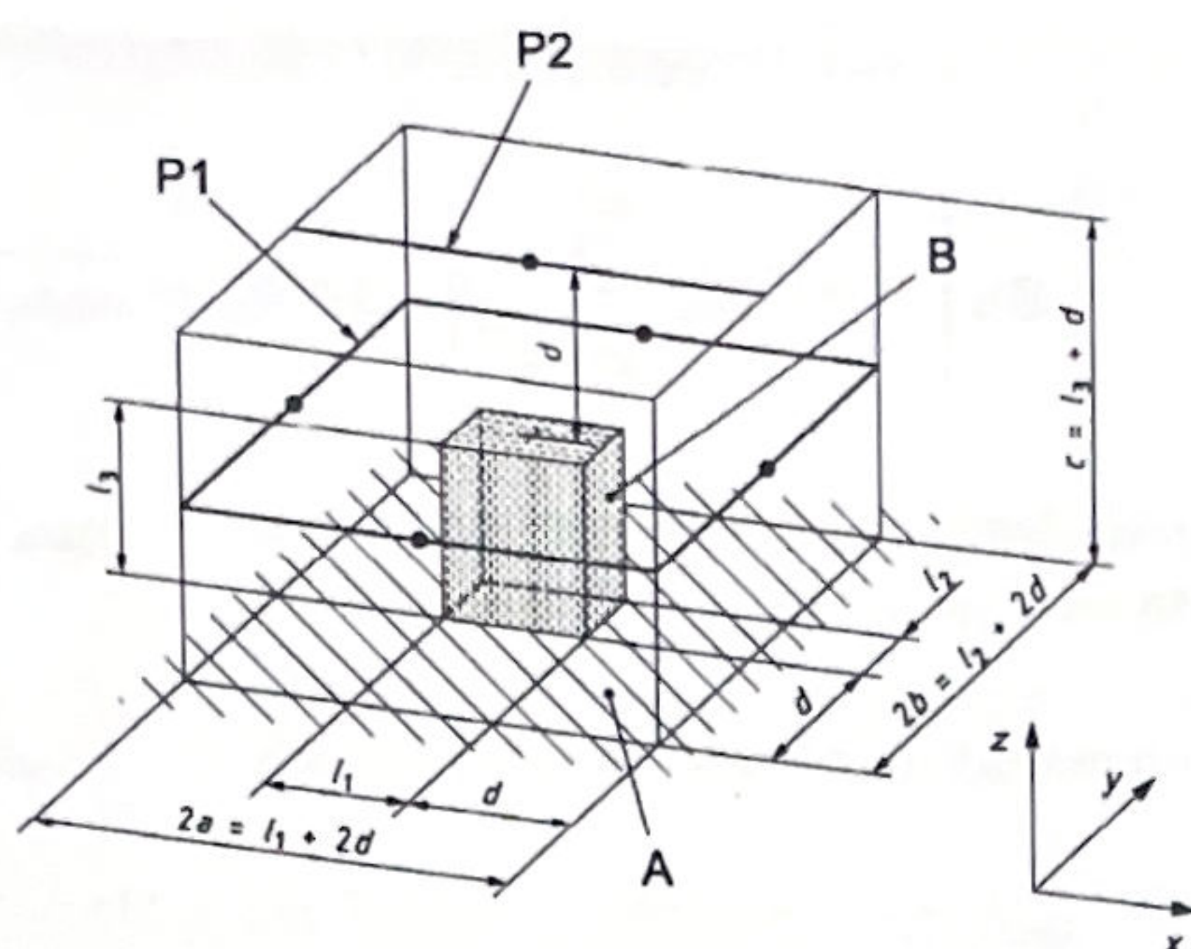
Abbildung 3: Messprinzip - quaderförmige Hüllfläche nach ÖNORM EN ISO 3746
