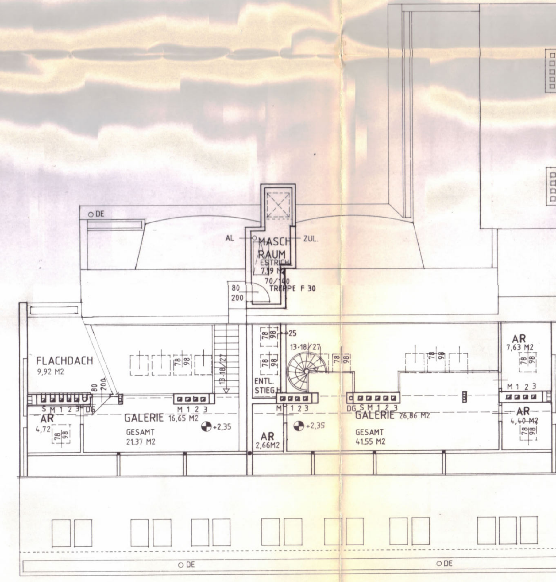
LUFTRAUM / GALERIE
