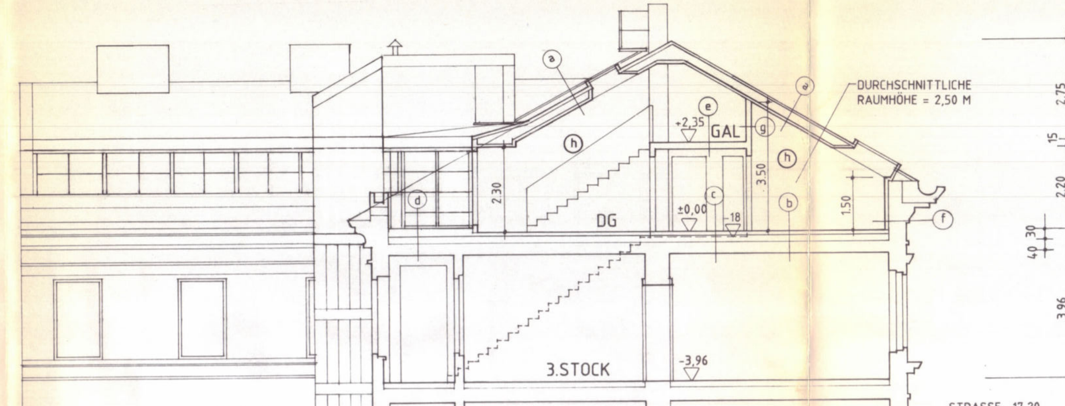
SNITT A-A
