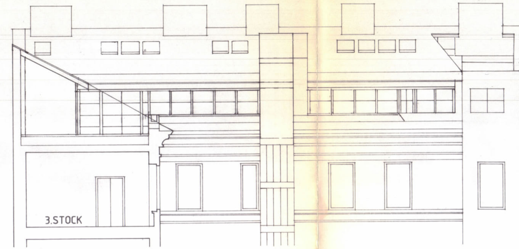
HOFANSICHT
