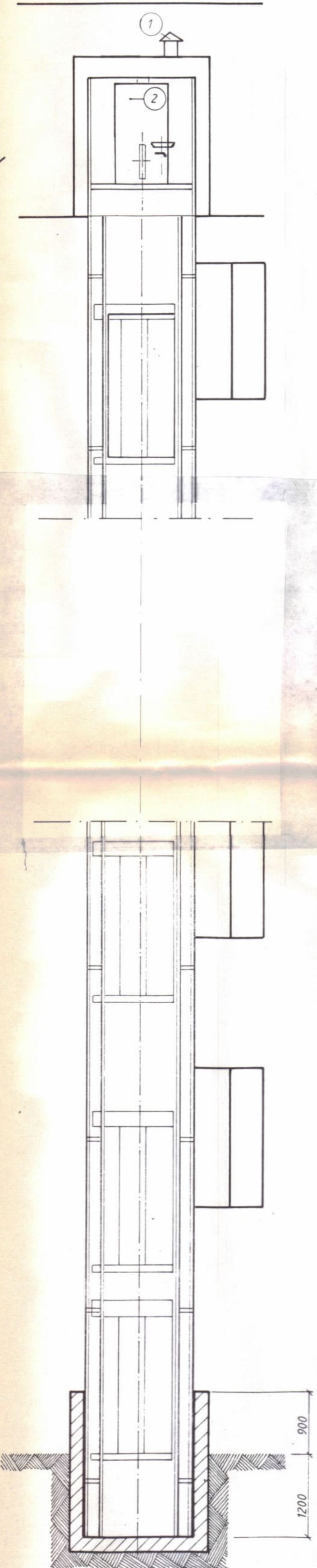
SCHNITT C-D M 1:50
