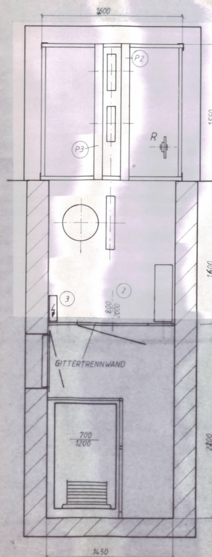
TWR-GRUNDRISS M 1:25 ZUGANG ÜBER DACHBODEN
