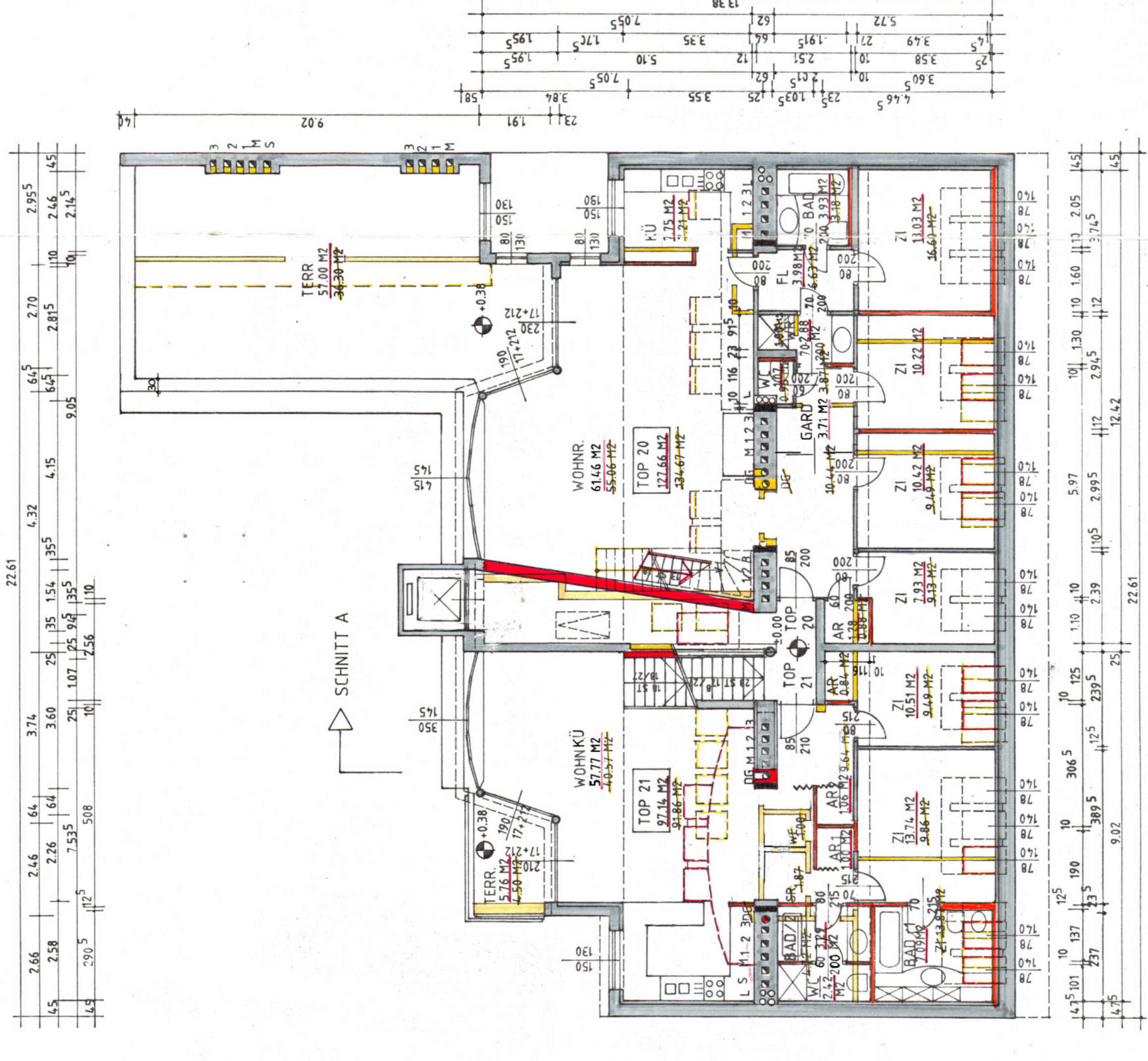
DACHGESCHOSS
