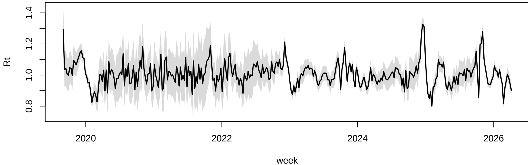
Rt: EpiEstim (Cori) vs SEIR-V2 \beta \cdot S/N
