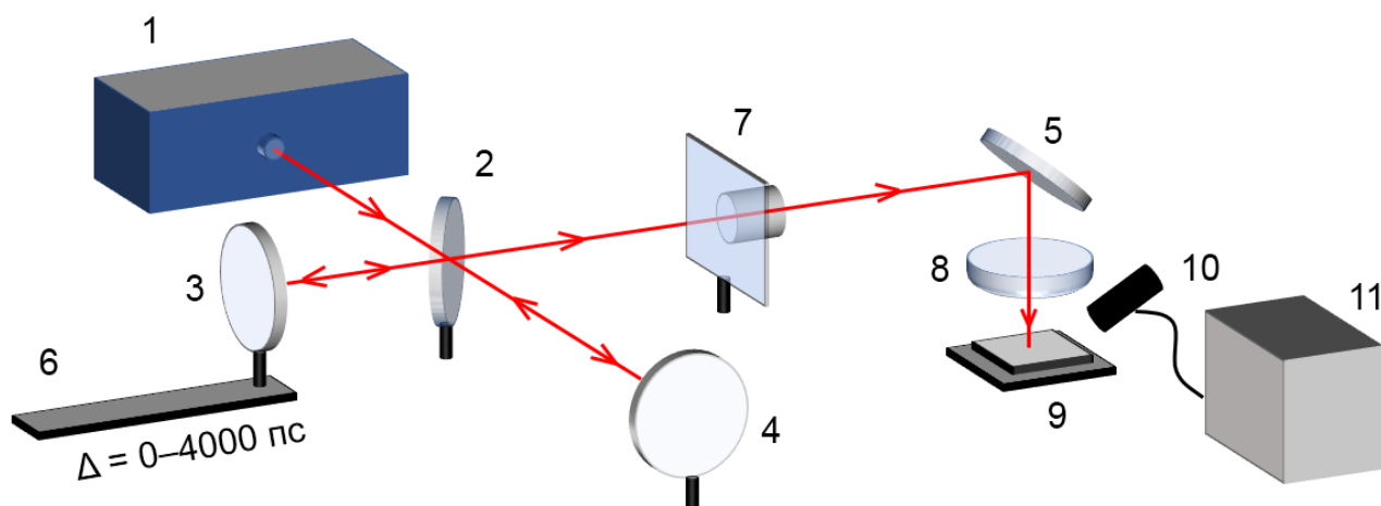
Рисунок 11. Оптическая схема эксперимента: 1 – лазерная система, 2 — полупрозрачное зеркало, 3, 4, 5 – зеркала, 6 – трансляционный столик, \Delta = 0\text{--}4000\text{ пс} , 7 – дифракционный ослабитель, 8 – собирающая линза, 9 – мишень, 10 – УЗ датчик, 11 – осциллограф.
