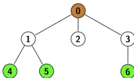
Ilustración 6 - Grafo acíclico
