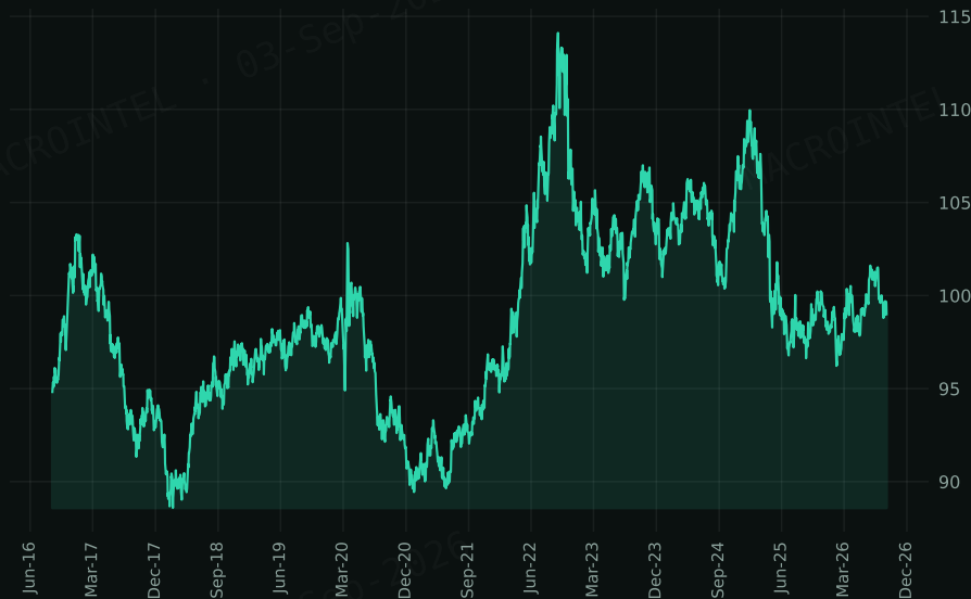
DXY · Spot
