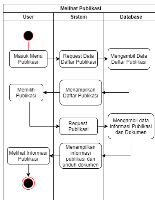
Gambar 7 User melihat publikasi
