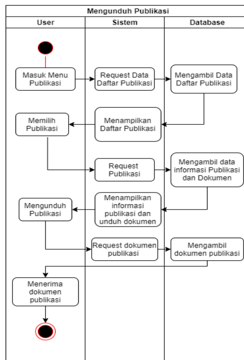
Gambar 3 User unduh publikasi
