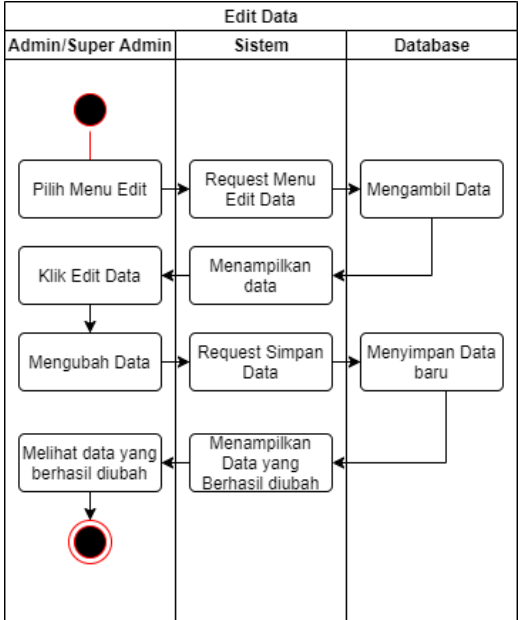
Gambar 15 Super admin/admin mengubah data foto, kampung, pengumuman, publikasi, video
