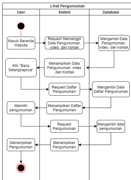
Gambar 8 User melihat pengumuman
