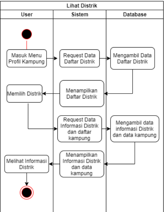
Gambar 13 User lihat distrik
