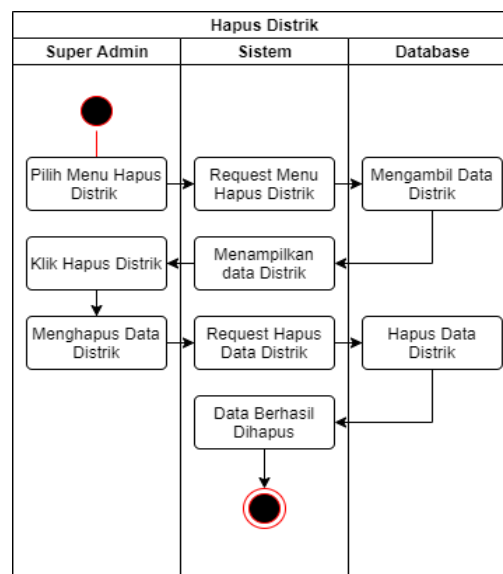
Gambar 10 Super admin menghapus distrik
