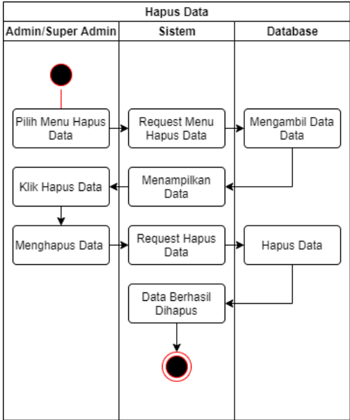
Gambar 14 Super admin/admin menghapus data foto, kampung, pengumuman, publikasi, video
