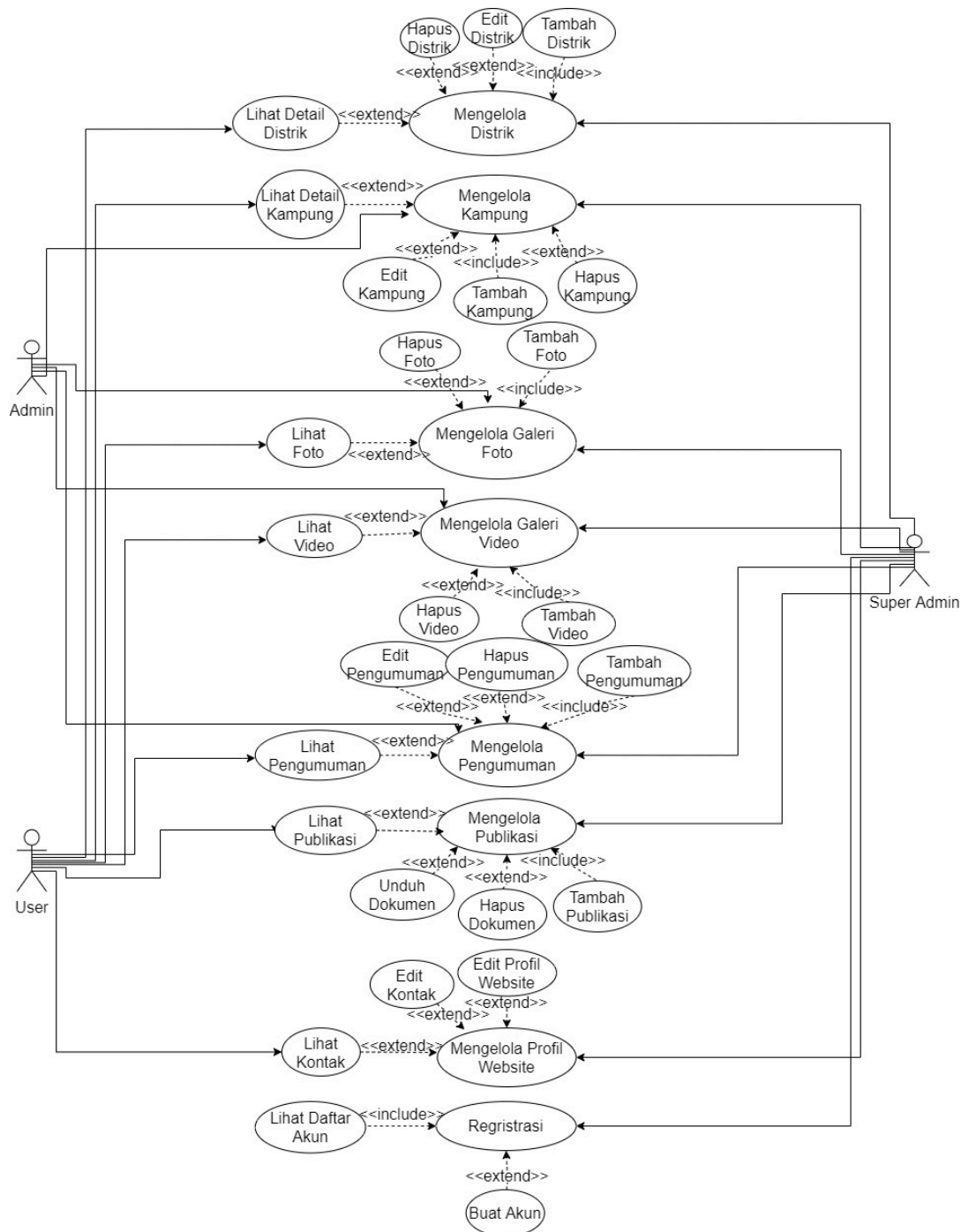
Gambar 2 Use case diagram website DPMPK Pegunungan Bintang
