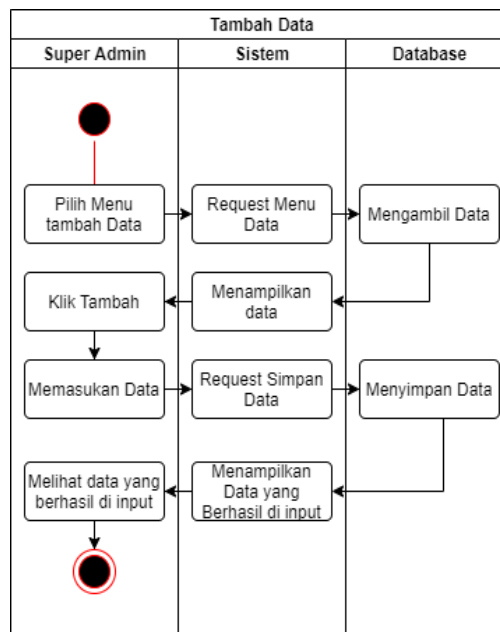
Gambar 6 Super admin tambah data akun dan distrik
