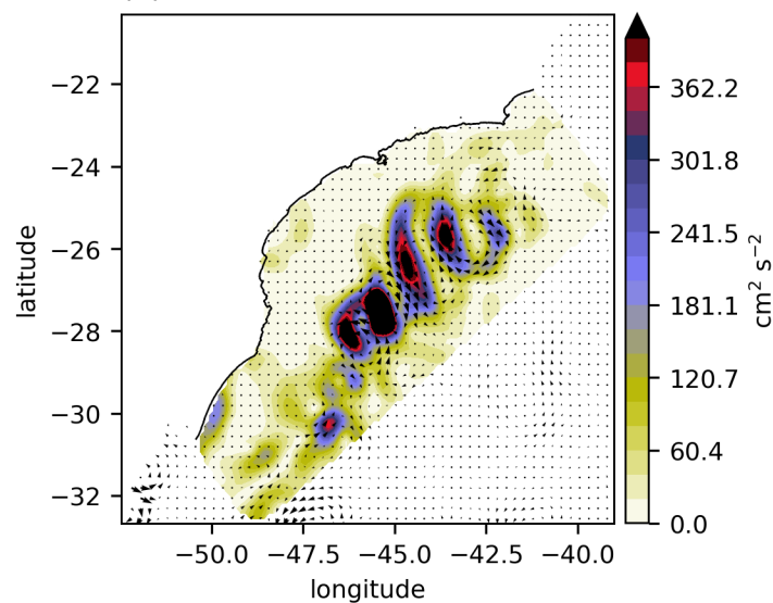
(d) altimetric surface EKE
