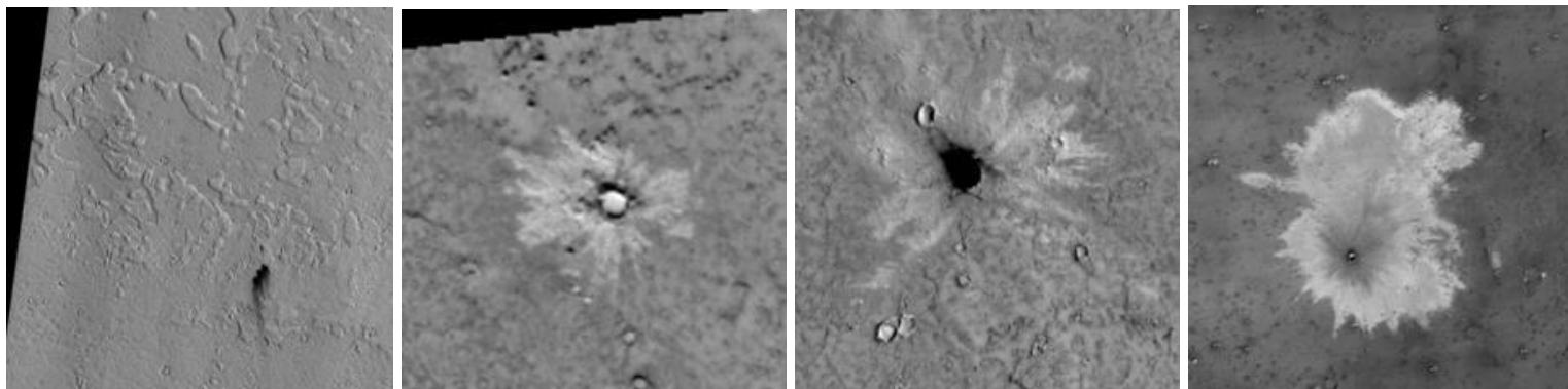
Impact Ejecta
