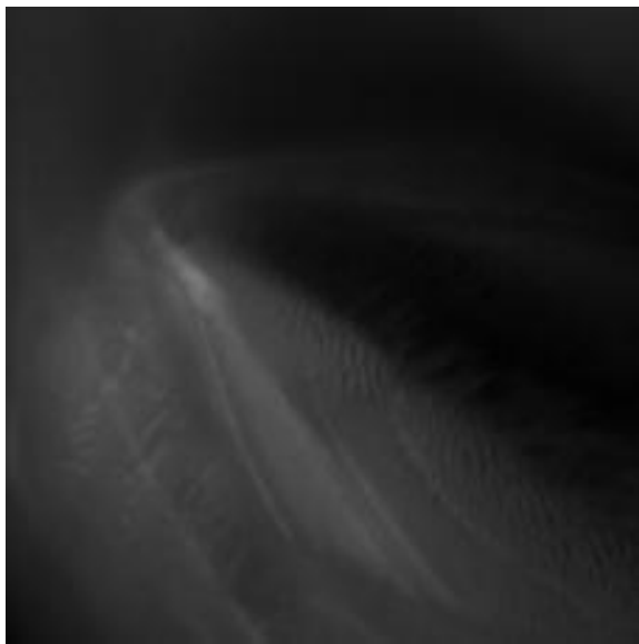
Dark Dune
