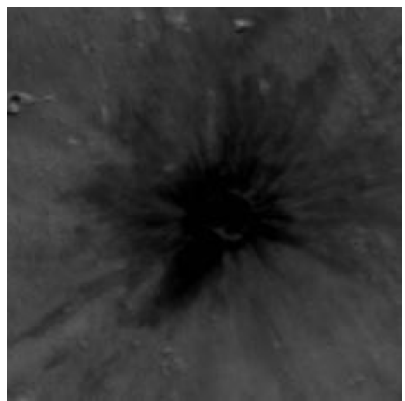
Impact Ejecta
