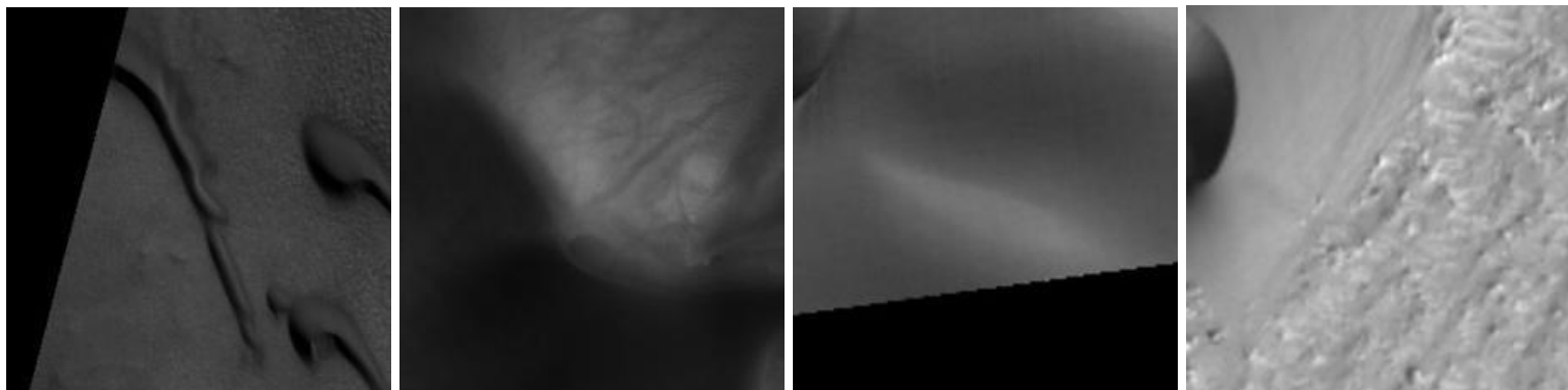
Impact Ejecta
