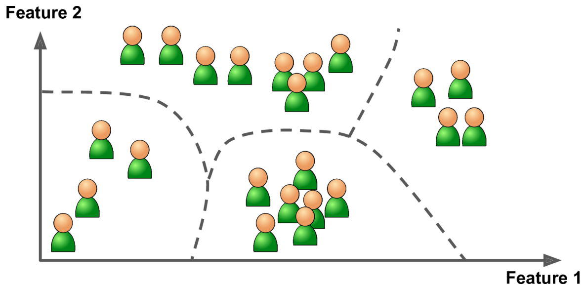
Figure 1-8. Clustering
