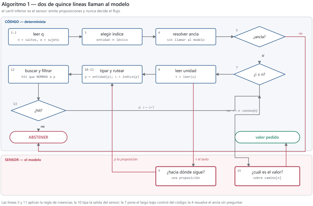
Flujo de control del Algoritmo 1
