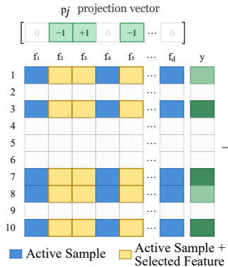
Dataset
