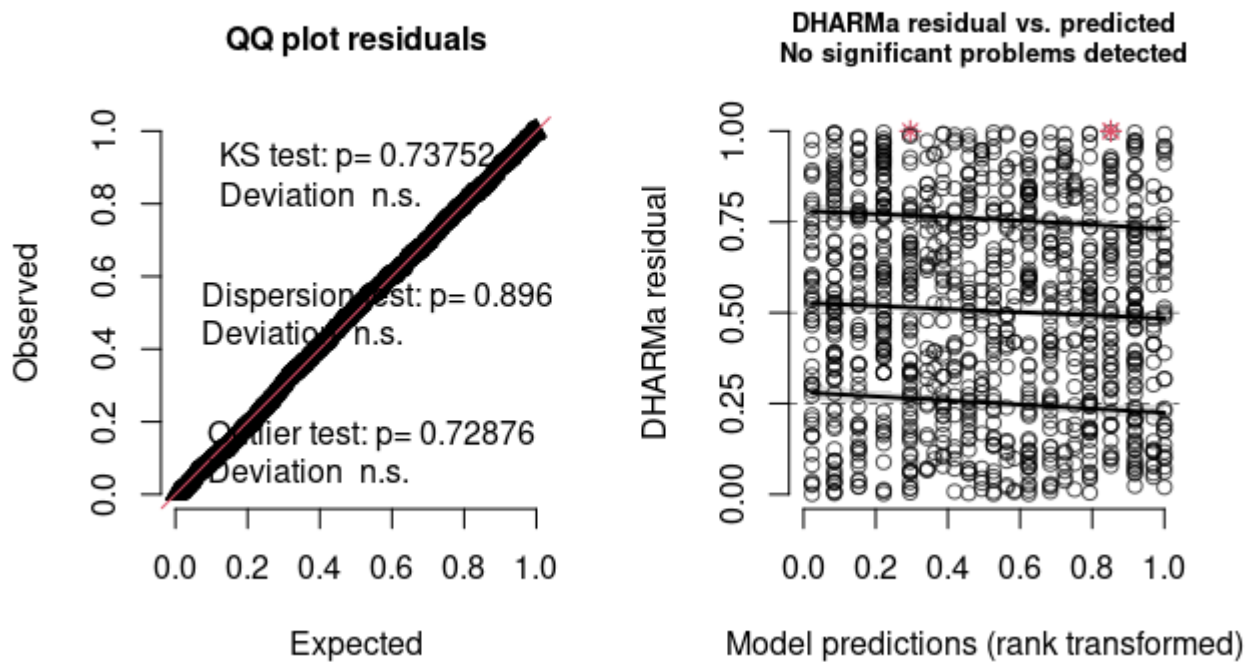
Figura 3: Diagnóstico con DHARMA del modelo macrohabitat de abundancia total
