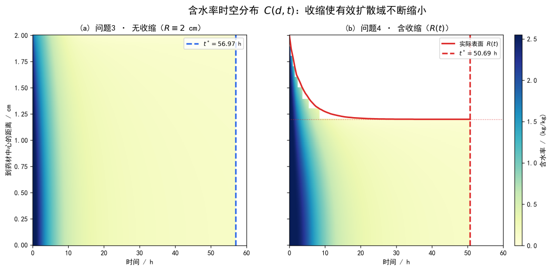
图 2: 问题 4 的收缩模型对应图：由式 (??)、(??)、(??) 及 R(t) 变动导致的含水率时空分布。该图体现收缩缩短扩散路径、加速干燥的机制。
