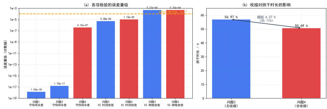
图 3: 模型验证与灵敏度分析：对应式 (17)、(20) 及仿真结果的收敛性、守恒性与参数敏感性检验
