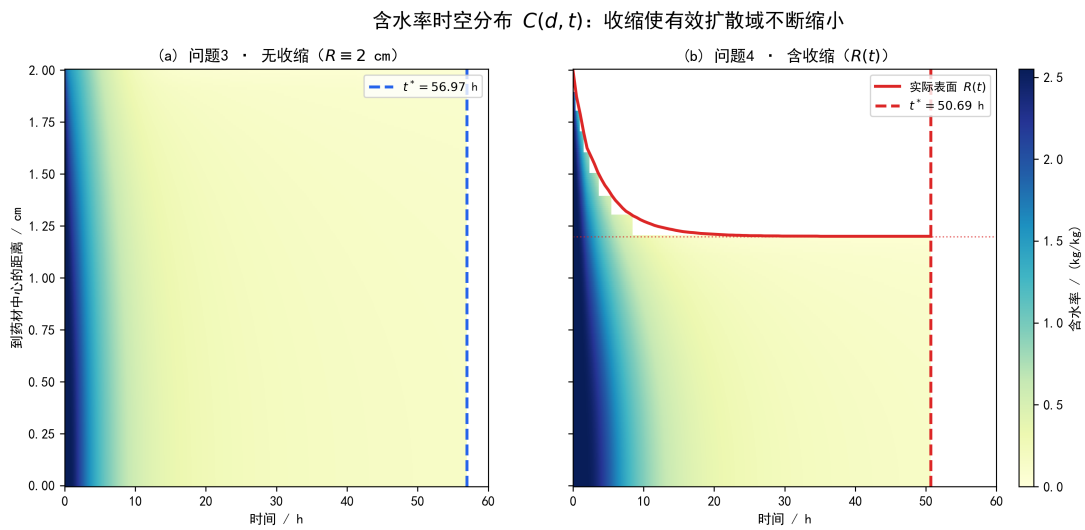
图 1: 问题 4 的收缩模型对应图：由式 (12)、(13)、(14) 及 R(t) 变动导致的含水率时空分布。该图体现收缩缩短扩散路径、加速干燥的机制。
