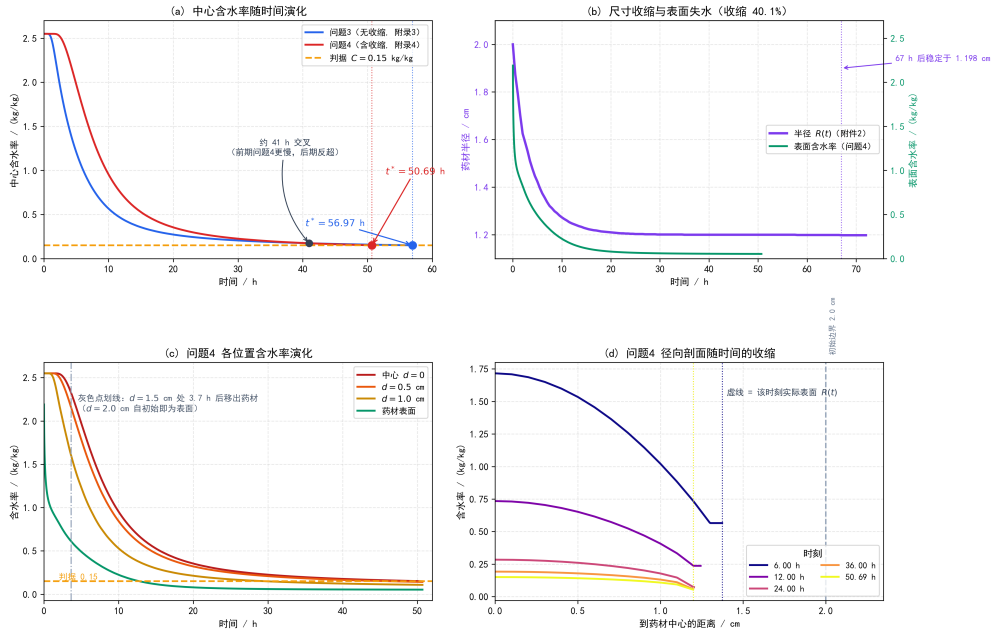
A题 药材烘干 · 含收缩前后对比总览
