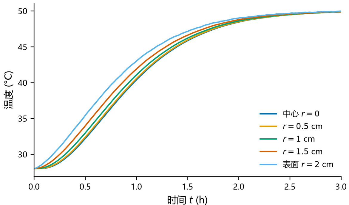
图 6: 问题 2 前 3 h 的温度演化：不同径向位置的温度随时间变化，反映了热扩散迅速达到近似均匀。
