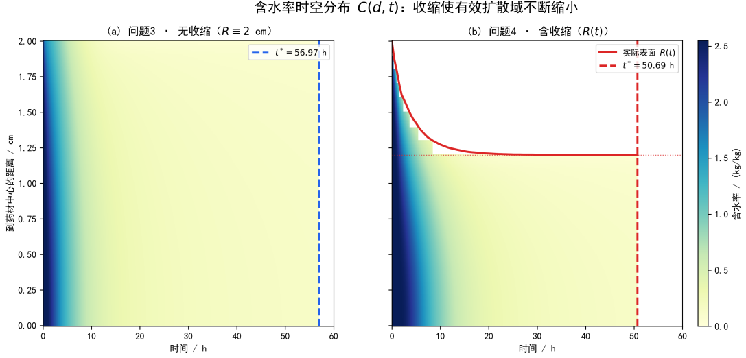
图 4: 问题 4 收缩模型下的含水率时空分布: 由式 (12)、(13)、(14) 与 R(t) 变动引起的干燥特征。
