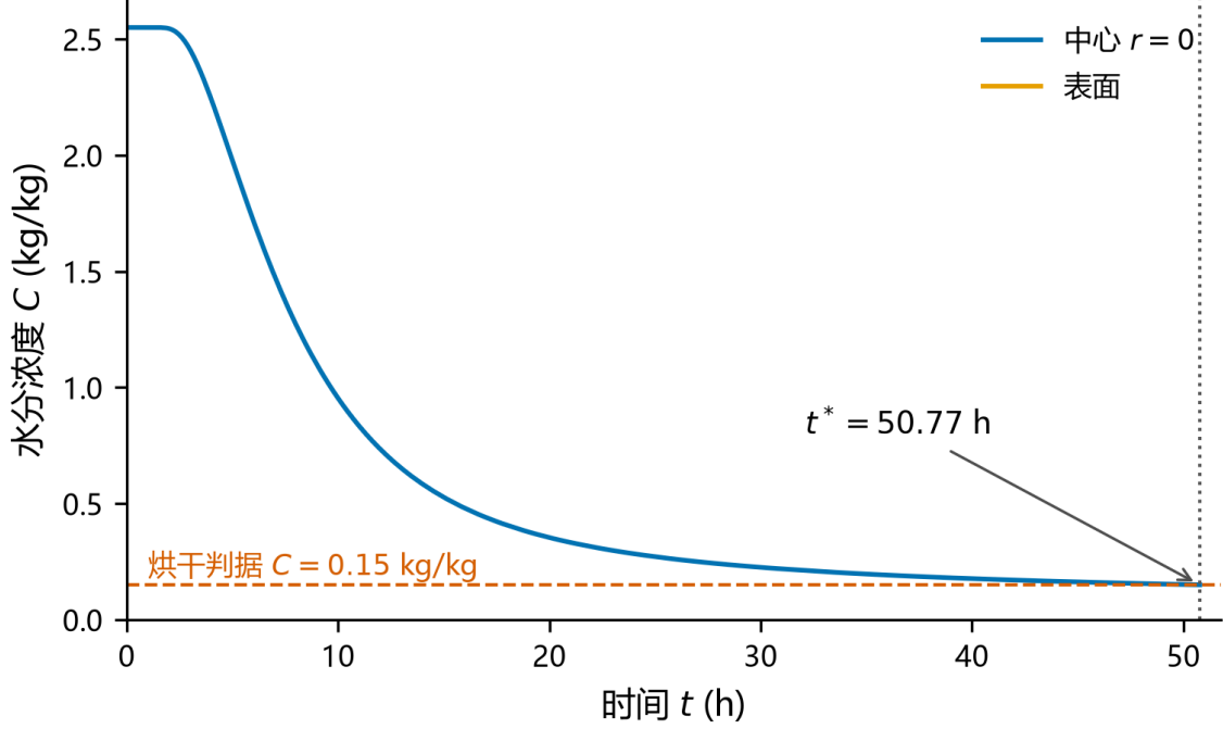
图 8: 问题 4 含收缩情况下的中心与表面含水率演化：收缩显著缩短扩散路径并提前达到烘干判据。
