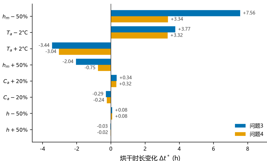
图 9: 参数灵敏度分析：烘房温度与传质系数变化对问题 3、4 烘干时长的影响。
