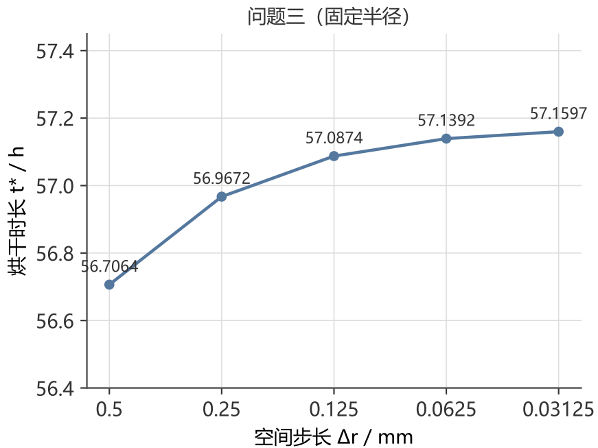
图 11 烘干时长 t^* 随空间网格加密的收敛情况
