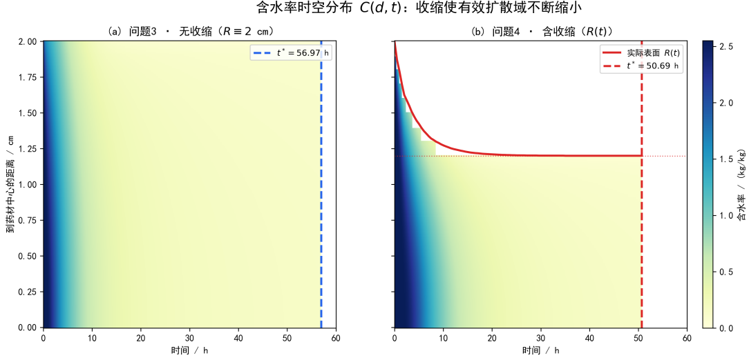
图 2: 问题 4 的收缩模型对应图: 由式 (12)、(13)、(14) 及 R(t) 变动导致的含水率时空分布。该图体现收缩缩短扩散路径、加速干燥的机制。
