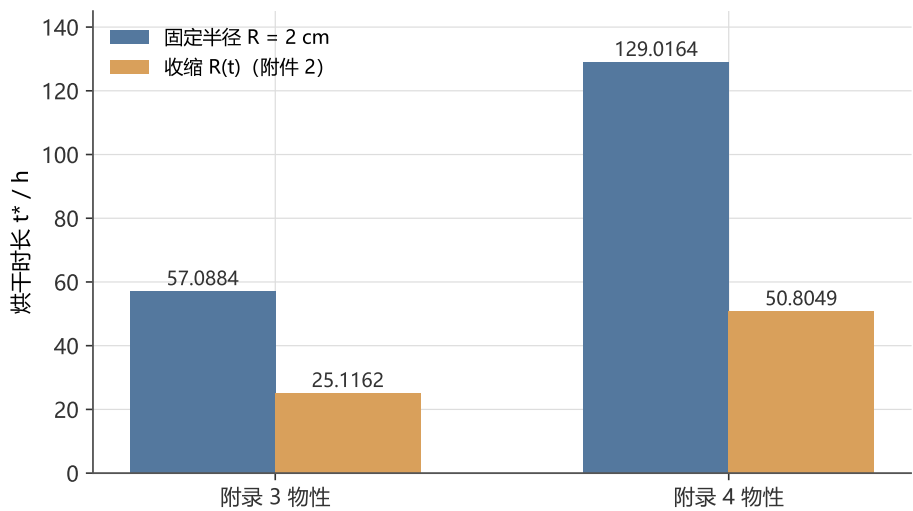
图 9 物性 \times 几何 2 \times 2 消融对照的烘干时长
