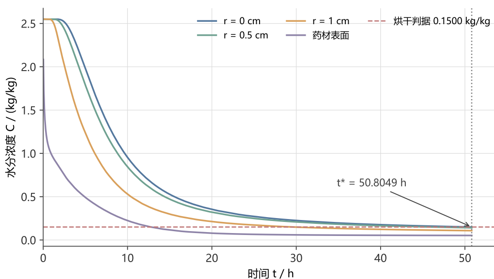
图 8 问题四含收缩药材水分浓度随时间的全程演化
