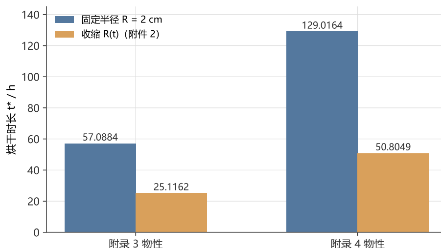
图 9 物性 × 几何 2×2 消融对照的烘干时长
