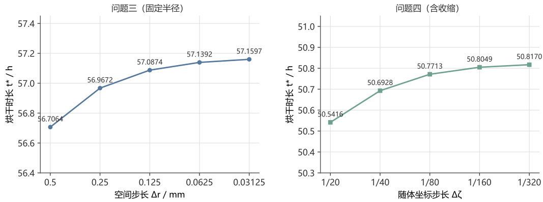
图 11 烘干时长 t^* 随空间网格加密的收敛情况
