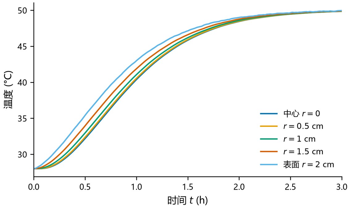
图 3: 问题 2 前 3 h 的温度演化：不同径向位置的温度随时间变化，体现双向耦合模型下热场达到近似均匀的过程。
