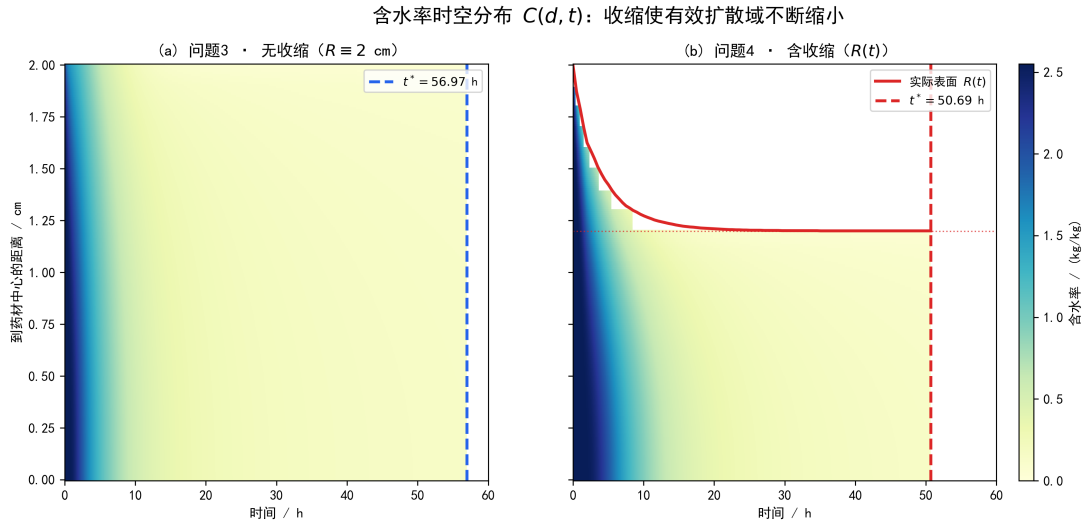
图 2: 问题 4 收缩模型下的含水率时空分布：由式 (12)、(13)、(14) 与 R(t) 变动引起的干燥特征。
