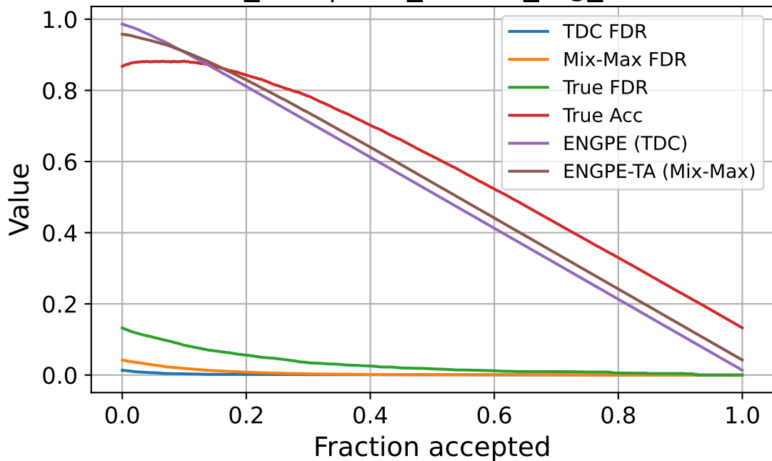
enc_256 | corr_source_fog_sev1
