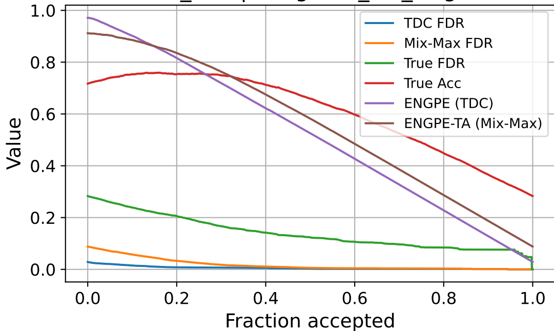
enc_256 | imagenet_val_target
