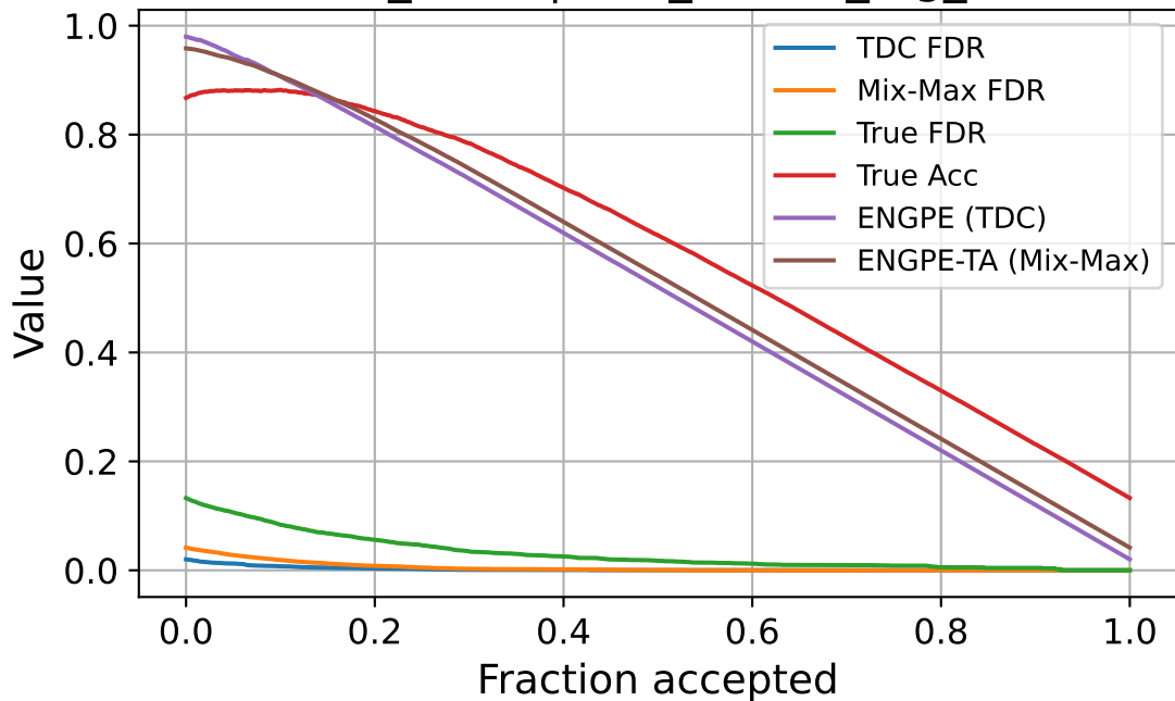
zscore_norm | corr_source_fog_sev1
