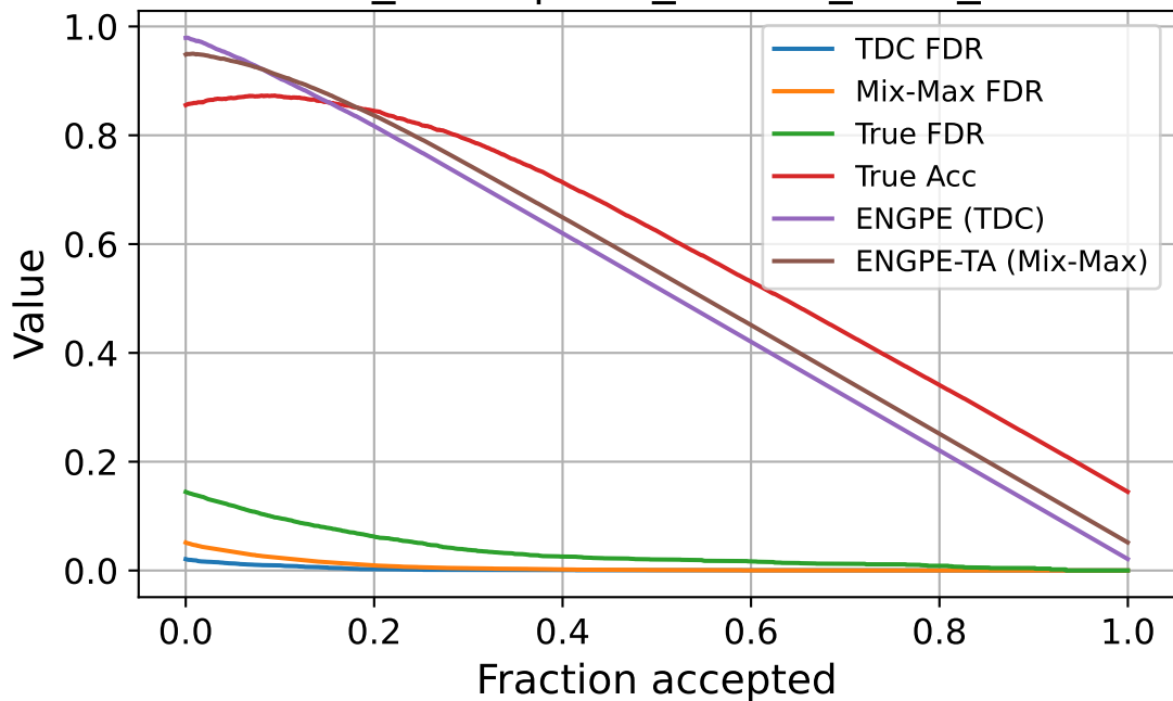
zscore_norm | corr_source_frost_sev1
