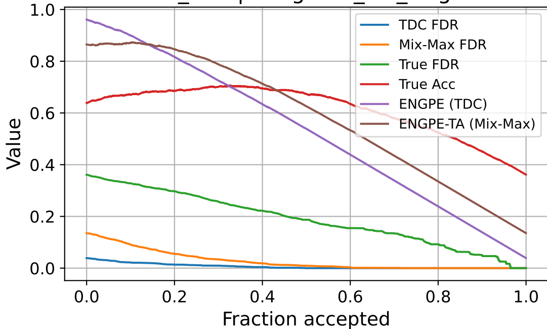
enc_256 | imagenet_val_target
