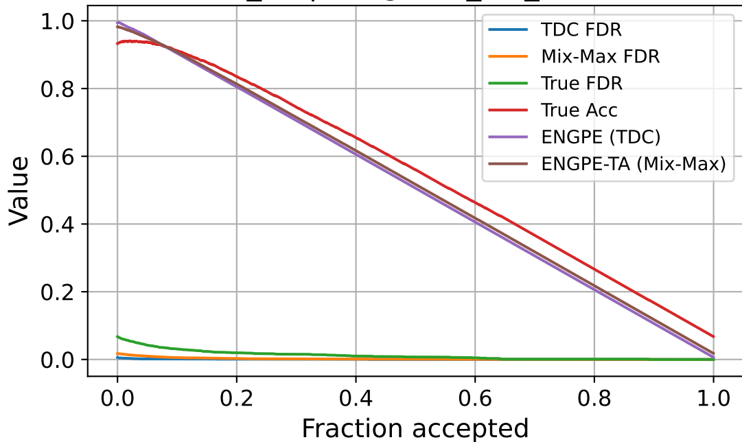
enc_64 | imagenet_val_source
