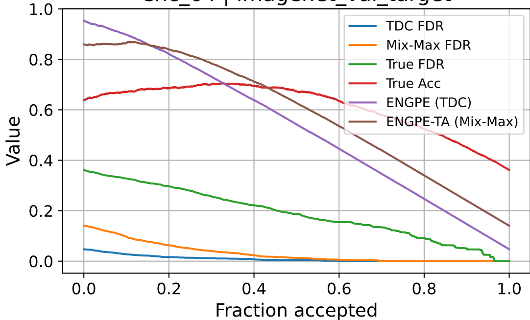
enc_64 | imagenet_val_target
