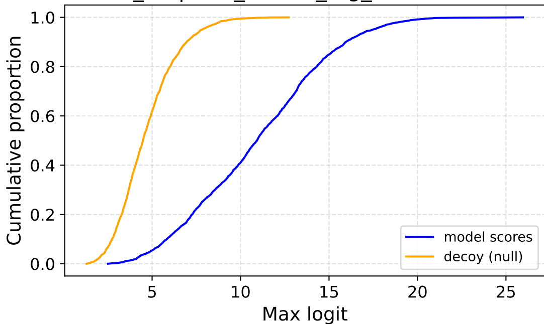
enc_64 | corr_source_fog_sev2 — ECDF
