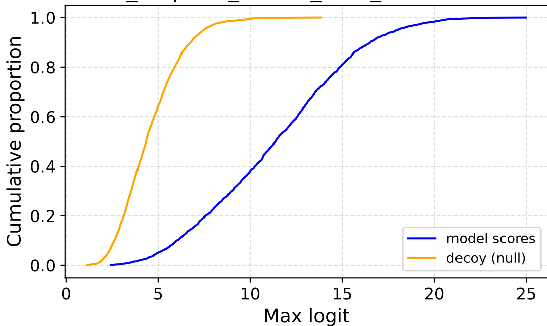
enc_64 | corr_source_frost_sev1 — ECDF
