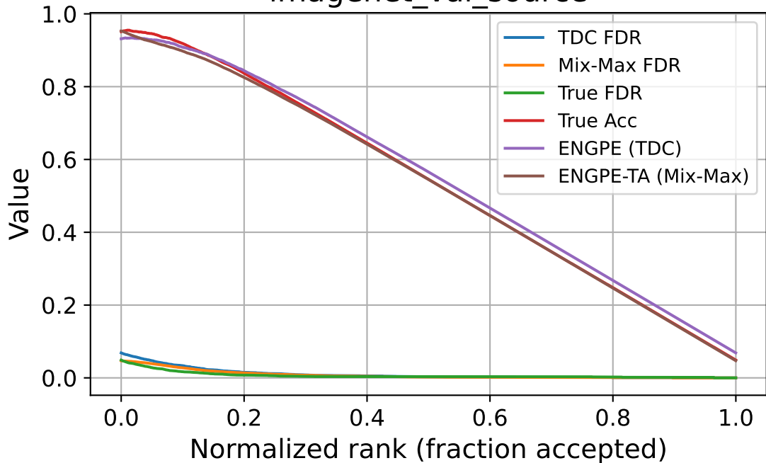
imagenet_val_source
