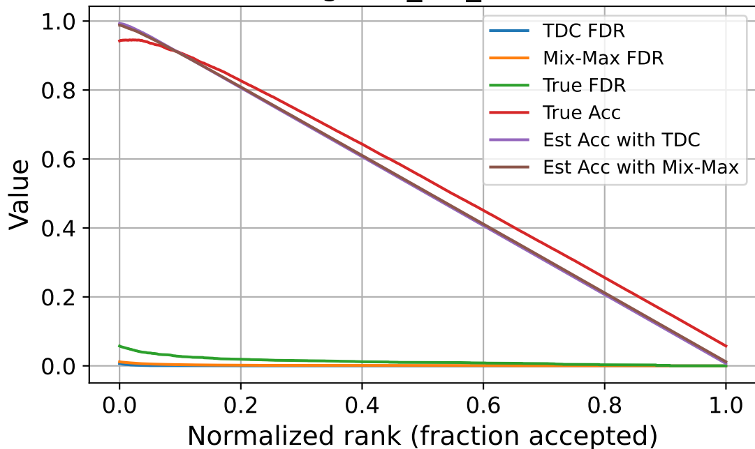
imagenet_val_source
