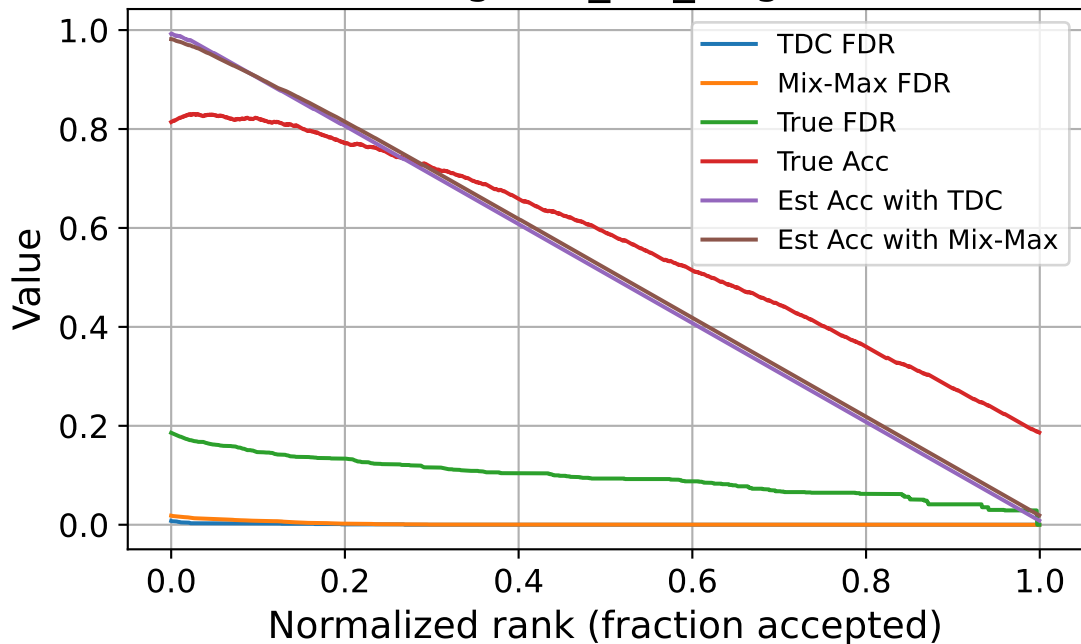
imagenet_val_target
